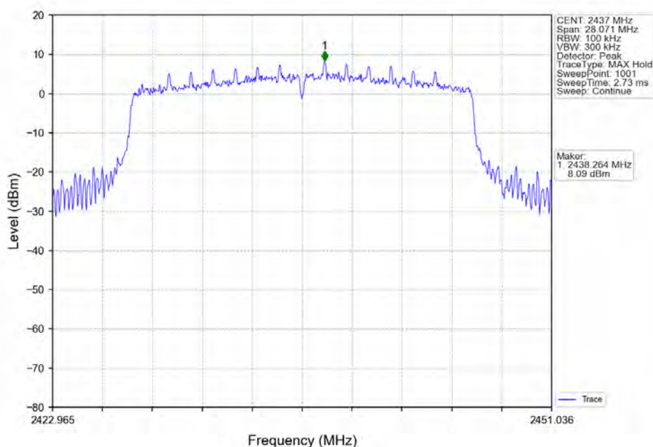
802.11ax(HE20)_MCH_2437MHz_RU242_Left_Ant2 (MIMO)_NTNV
