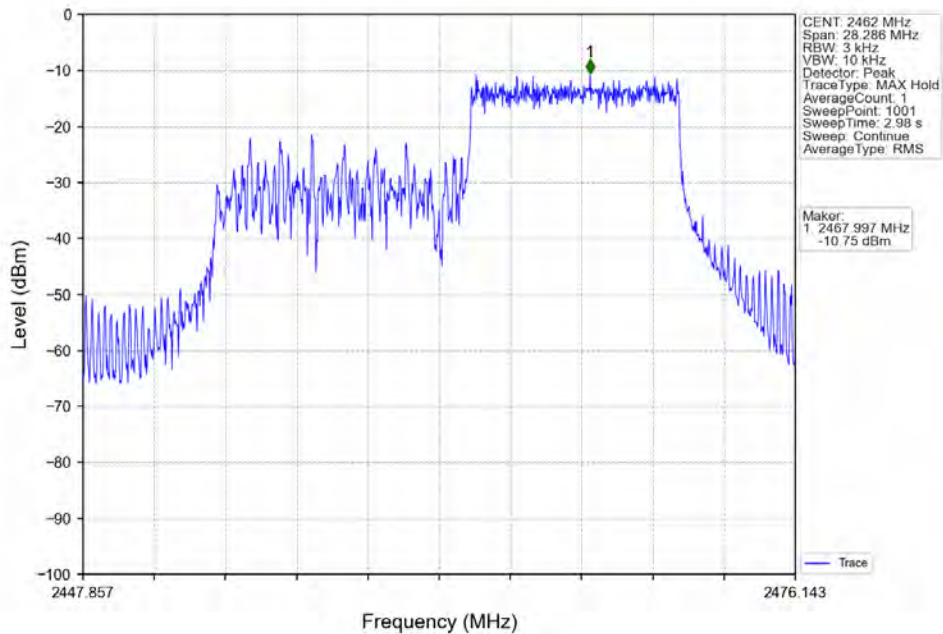
802.11ax(HE20)_HCH_2462MHz_RU106_Right_Ant1 (MIMO)_NTNV
