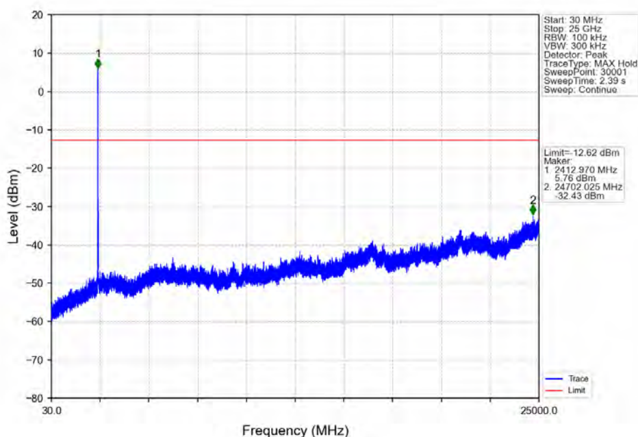
802.11ax(HE20) LCH 2412MHz RU242 Left Ant1 (MIMO) NTN
