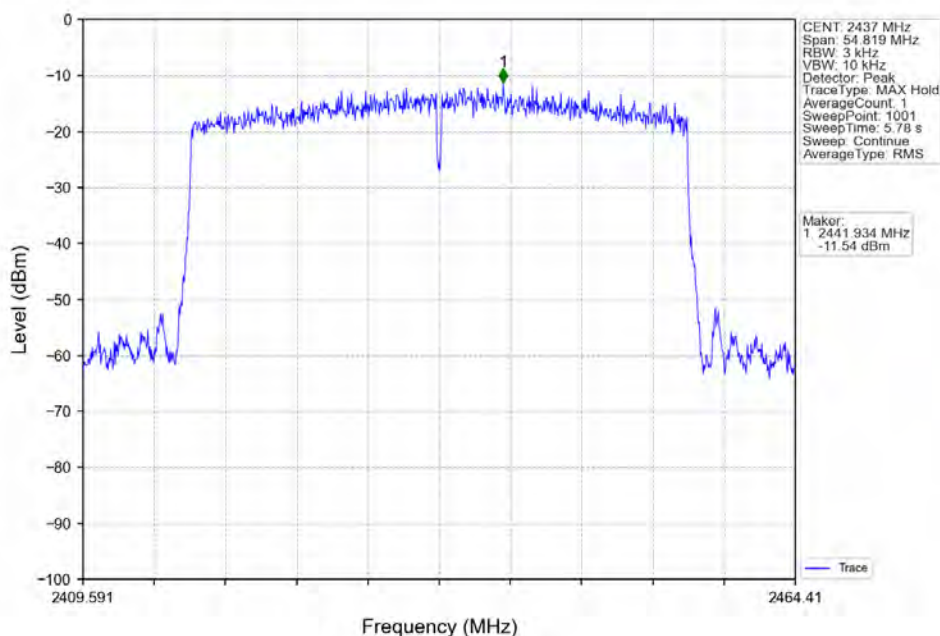
802.11ax(HE40)_MCH_2437MHz_RU484_Left_Ant1 (MIMO)_NTNV
