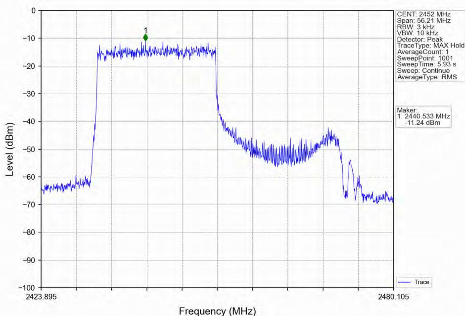
802.11ax(HE40)_HCH_2452MHz_RU242_Right_Ant1 (MIMO)_NTNV
