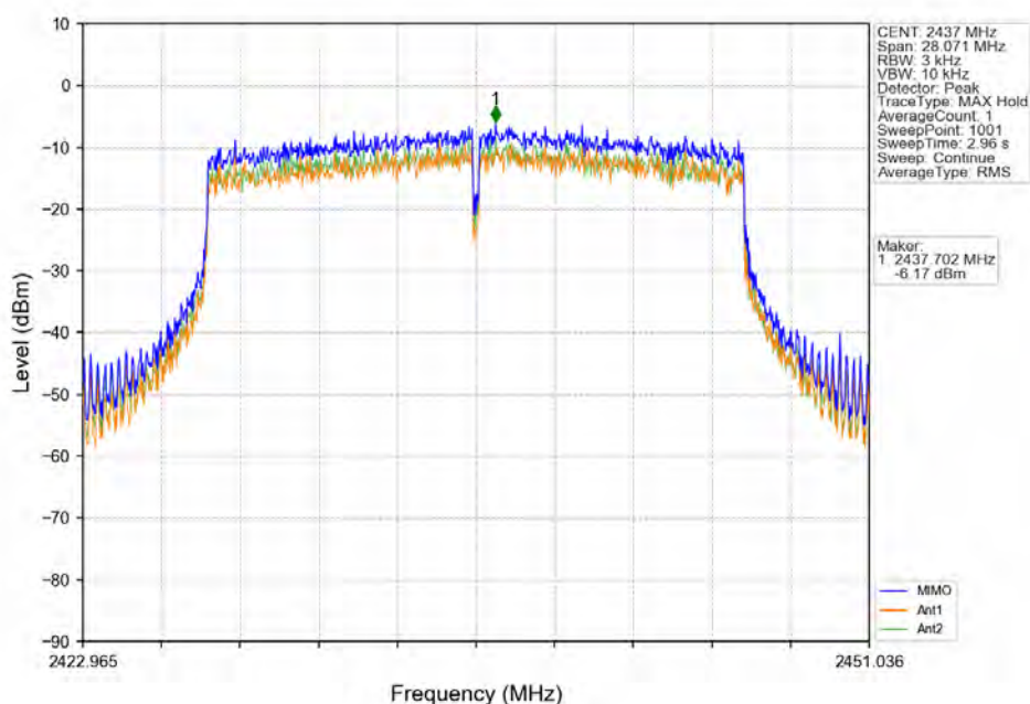
802.11ax(HE20)_MCH_2437MHz_RU242_Left_MIMO_NTNV
