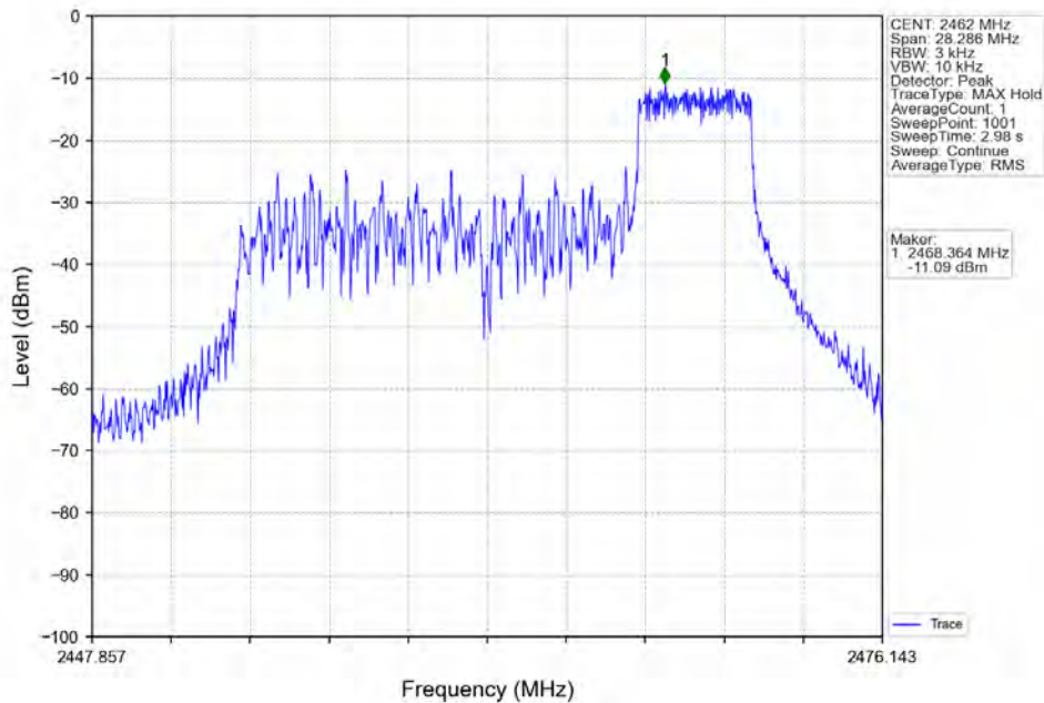
802.11ax(HE20)_HCH_2462MHz_RU52_Right_Ant1(MIMO)_NTNV
