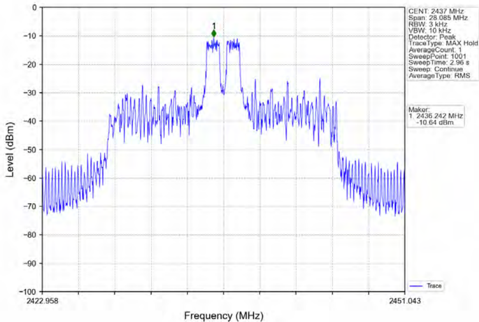
802.11ax(HE20)_MCH_2437MHz_RU26_Mid_Ant1 (MIMO)_NTNV
