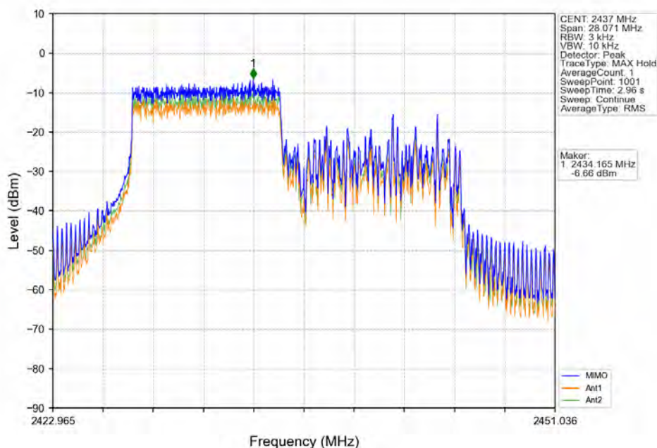
802.11ax(HE20)_MCH_2437MHz_RU106_Left_MIMO_NTNV
