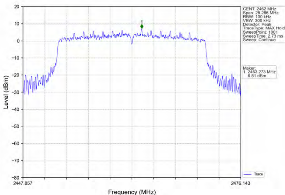
802.11ax(HE20)_HCH_2462MHz_RU242_Left_Ant1 (MIMO)_NTNV
