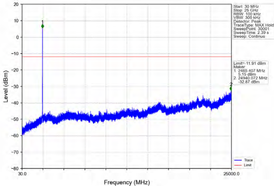
802.11ax(HE20)_HCH_2462MHz_RU242_Left_Ant2 (MIMO)_NTNV
