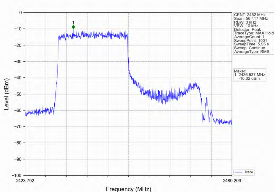
802.11ax(HE40)_HCH_2452MHz_RU242_Right_Ant2 (MIMO)_NTNV
