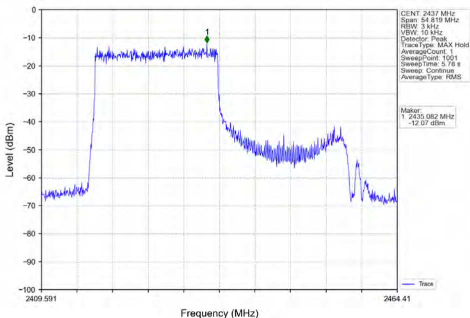
802.11ax(HE40)_MCH_2437MHz_RU242_Left_Ant1(MIMO)_NTNV
