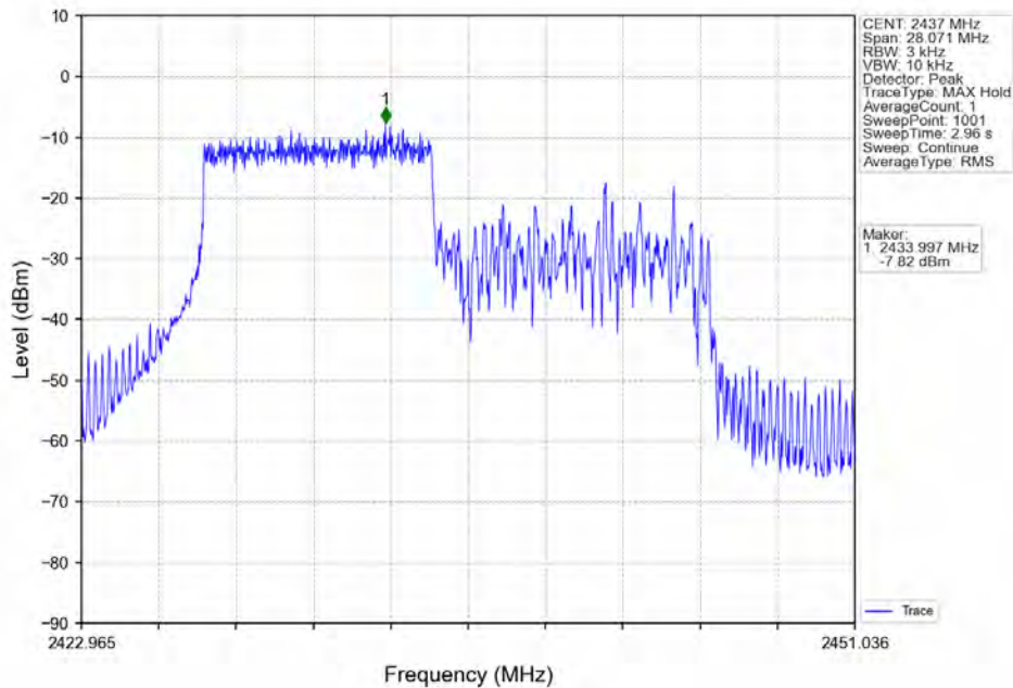
802.11ax(HE20)_MCH_2437MHz_RU106_Left_Ant2 (MIMO)_NTNV
