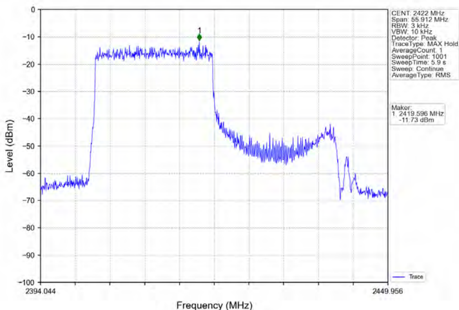
802.11ax(HE40) LCH 2422MHz RU242 Left Ant1 (MIMO) NTN
