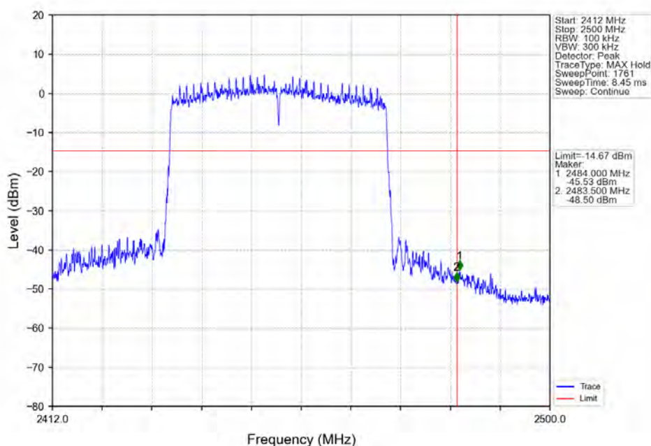
802.11ax(HE40)_HCH_2452MHz_RU484_Left_Ant2 (MIMO)_NTNV
