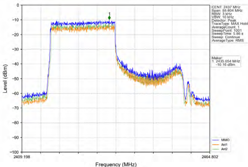
802.11ax(HE40)_MCH_2437MHz_RU242_Left_MIMO_NTNV
