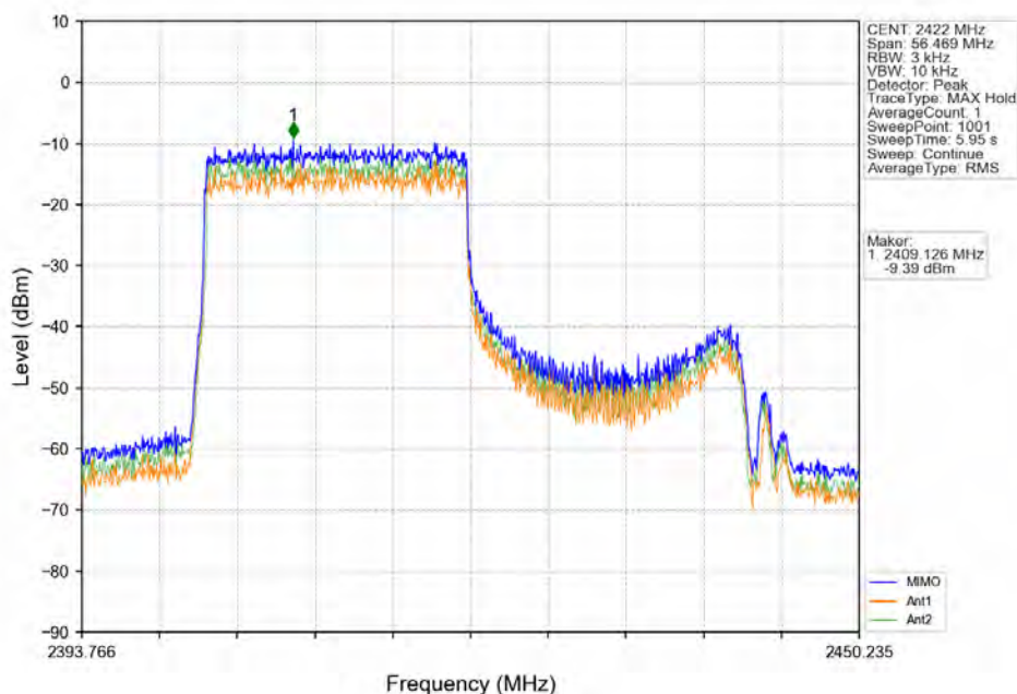
802.11ax(HE40) LCH_2422MHz_RU242_Left_MIMO_NTNV
