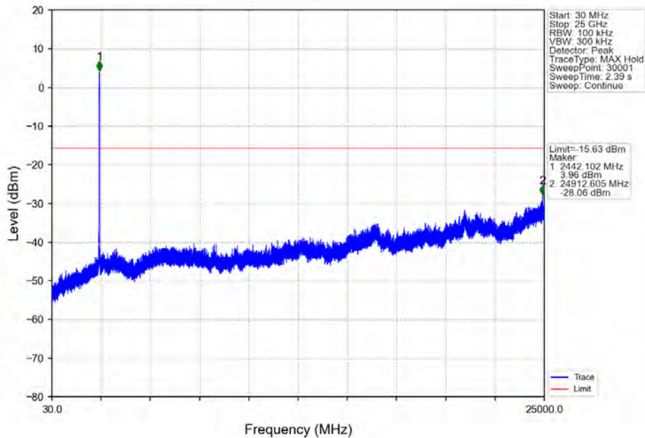
802.11ax(HE40)_MCH_2437MHz_RU484_Left_Ant1(MIMO)_NTNV
