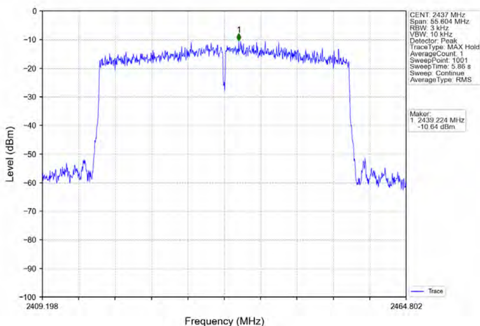
802.11ax(HE40)_MCH_2437MHz_RU484_Left_Ant2 (MIMO)_NTNV
