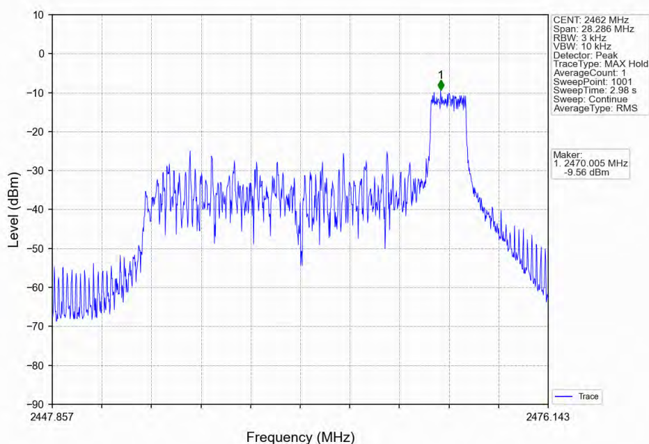
802.11ax(HE20)_HCH_2462MHz_RU26_Right_Ant1(MIMO)_NTNV
