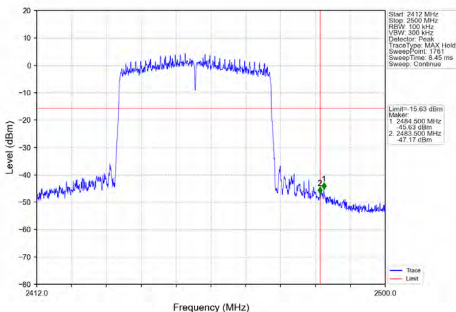
802.11ax(HE40)_HCH_2452MHz_RU484_Left_Ant1 (MIMO)_NTNV
