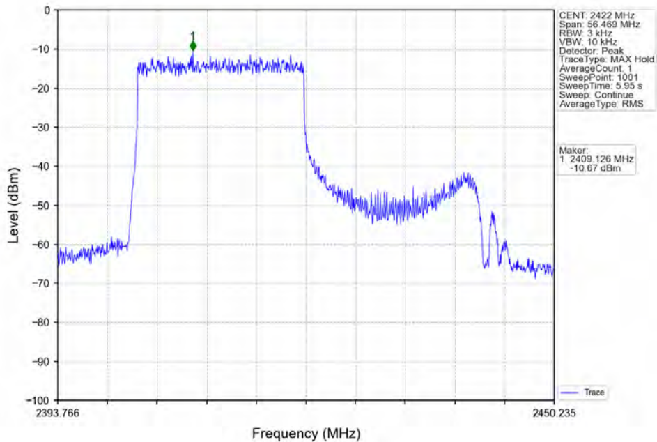
802.11ax(HE40) LCH 2422MHz RU242 Left Ant2 (MIMO) NTN
