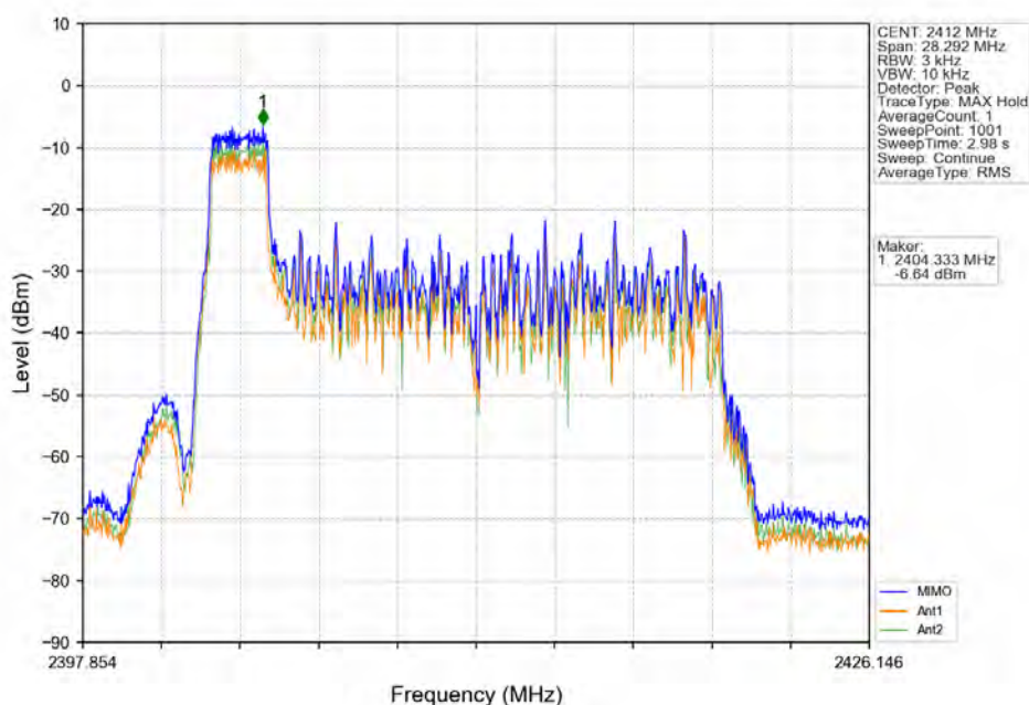
802.11ax(HE20)_LCH_2412MHz_RU26_Left MIMO_NTNV
