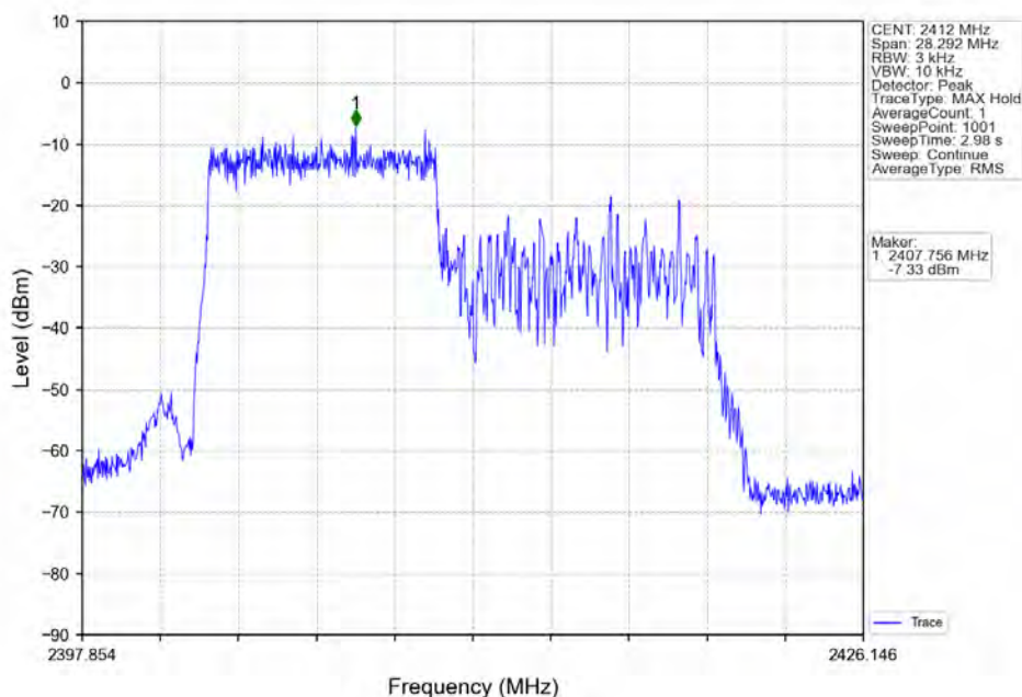
802.11ax(HE20) LCH 2412MHz RU106 Left Ant2 (MIMO) NTN
