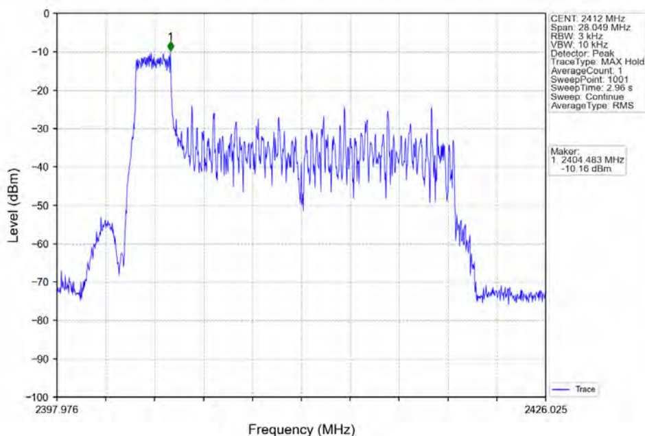
802.11ax(HE20)_LCH_2412MHz_RU26_Left_Ant1 (MIMO)_NTNV
