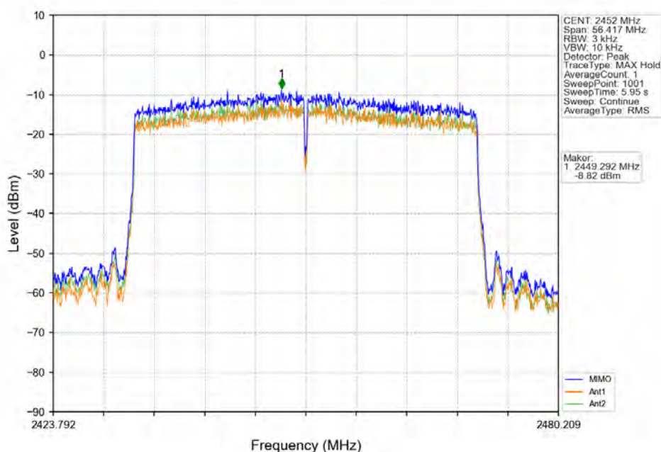
802.11ax(HE40)_HCH_2452MHz_RU484_Left_MIMO_NTNV
