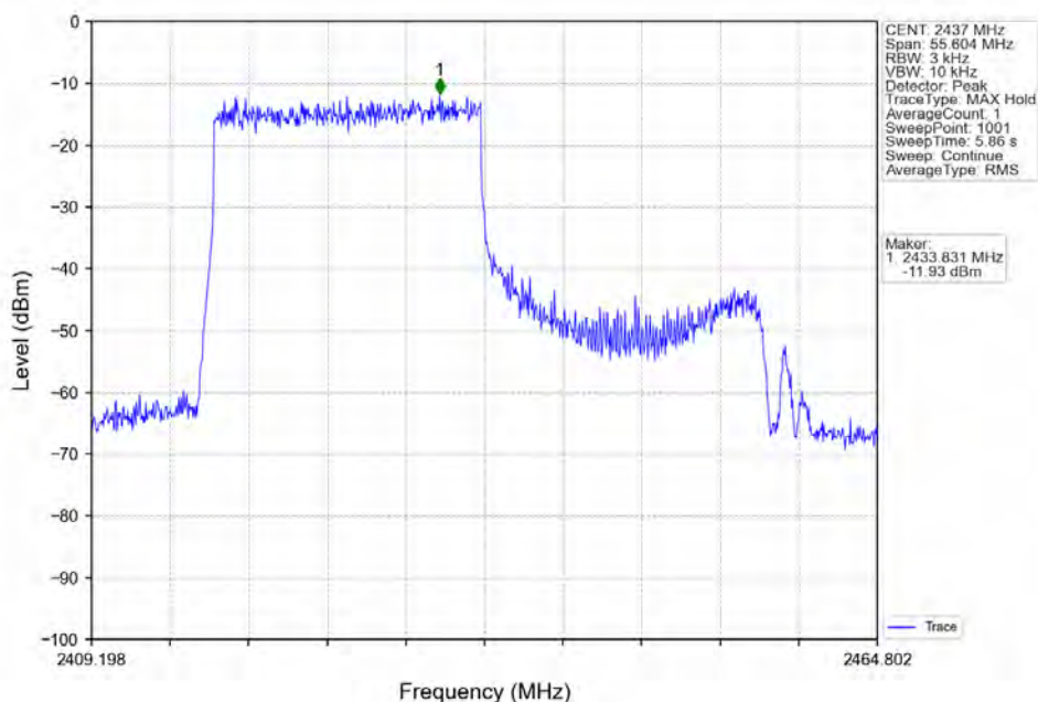
802.11ax(HE40)_MCH_2437MHz_RU242_Left_Ant2 (MIMO)_NTNV
