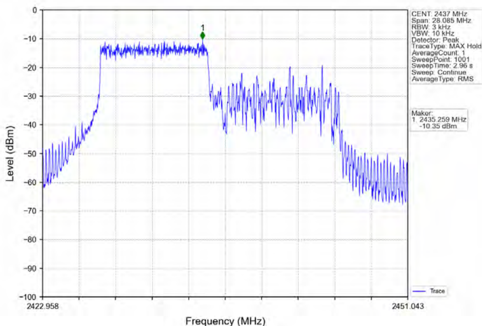
802.11ax(HE20)_MCH_2437MHz_RU106_Left_Ant1 (MIMO)_NTNV
