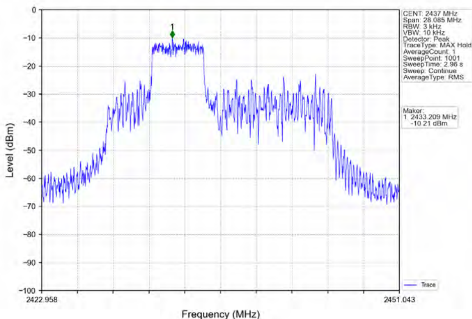
802.11ax(HE20)_MCH_2437MHz_RU52_Mid_Ant1 (MIMO)_NTNV
