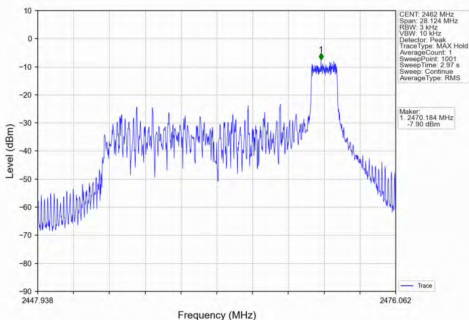
802.11ax(HE20)_HCH_2462MHz_RU26_Right_Ant2(MIMO)_NTNV
