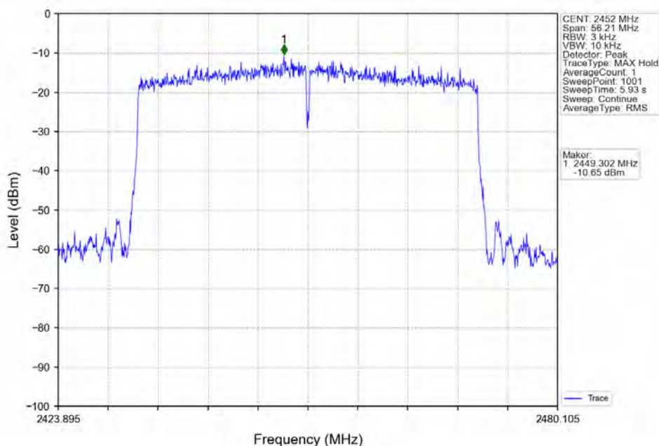
802.11ax(HE40)_HCH_2452MHz_RU484_Left_Ant1 (MIMO)_NTNV
