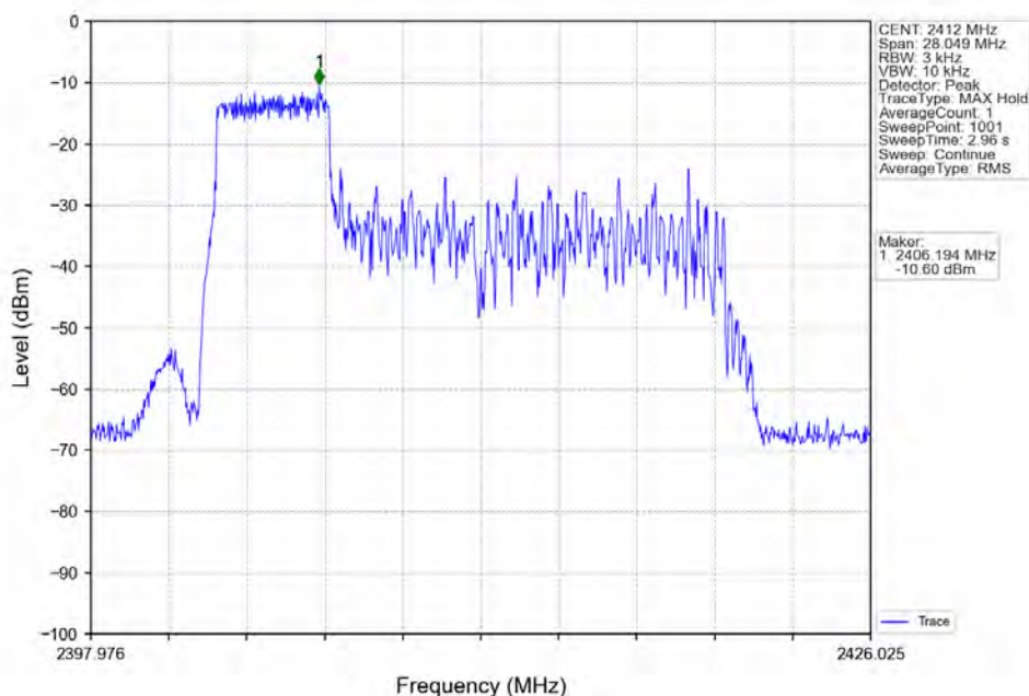
802.11ax(HE20)_LCH_2412MHz_RU52_Left_Ant1 (MIMO)_NTNV
