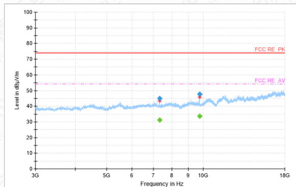
RSE-11N-CH6-3GHz-18GHz
