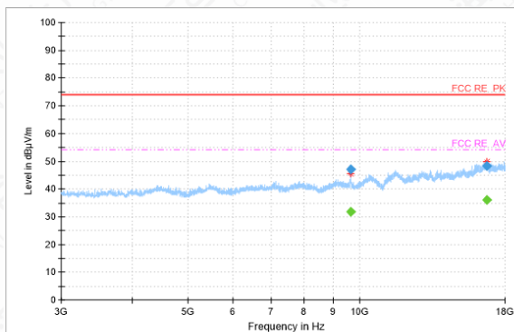
RSE-11N-CH1-3GHz-18GHz
