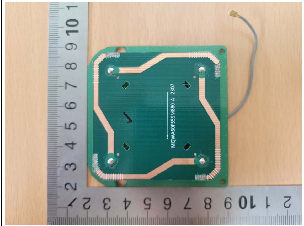
RFID Antenna
