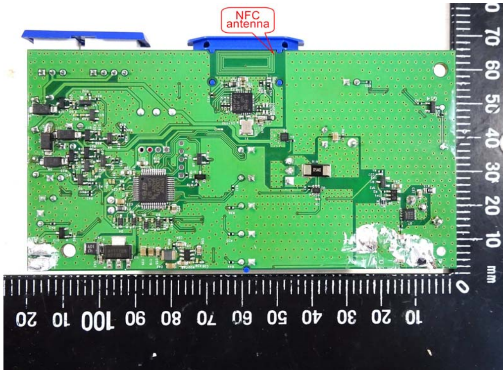
Antenna
