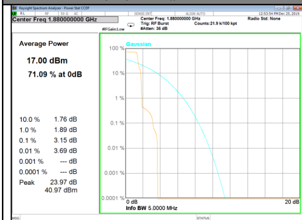
Band 2-15KHz-1#0-BPSK-Mid
