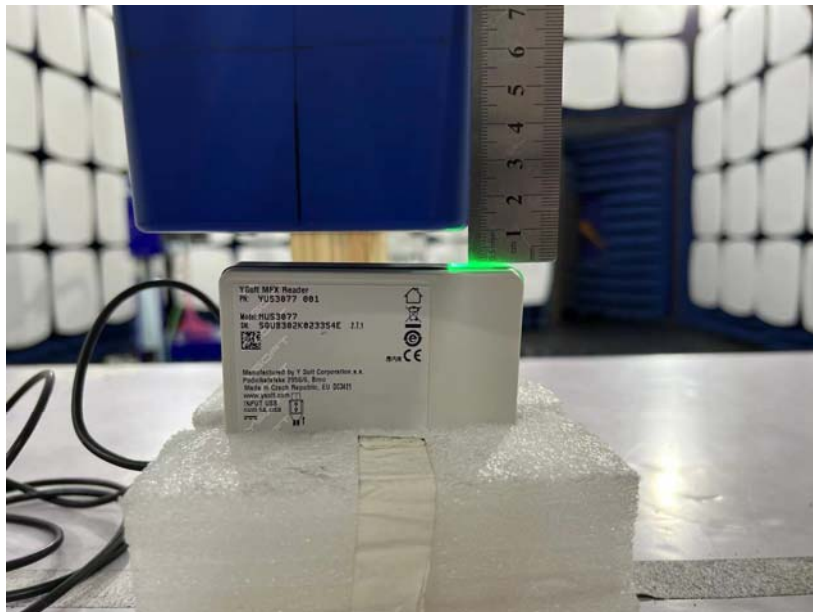
Bottom Side_10mm
