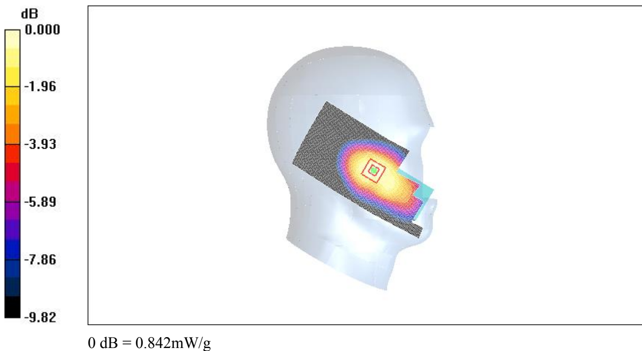
Fig. 3 850 MHz CH190
