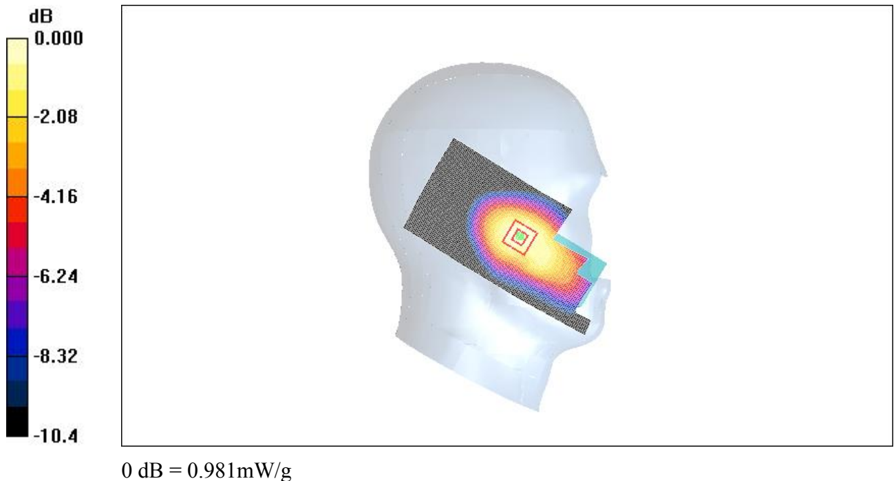
Fig. 1 850MHz CH251
