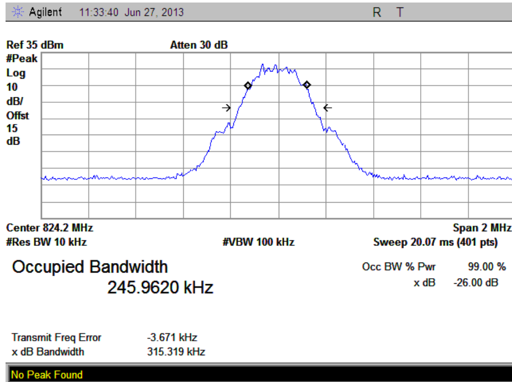
(Plot A: GPRS 850MHz Channel = 128)
