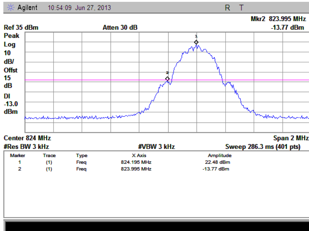
(Plot A: GPRS 850 Channel = 128)
