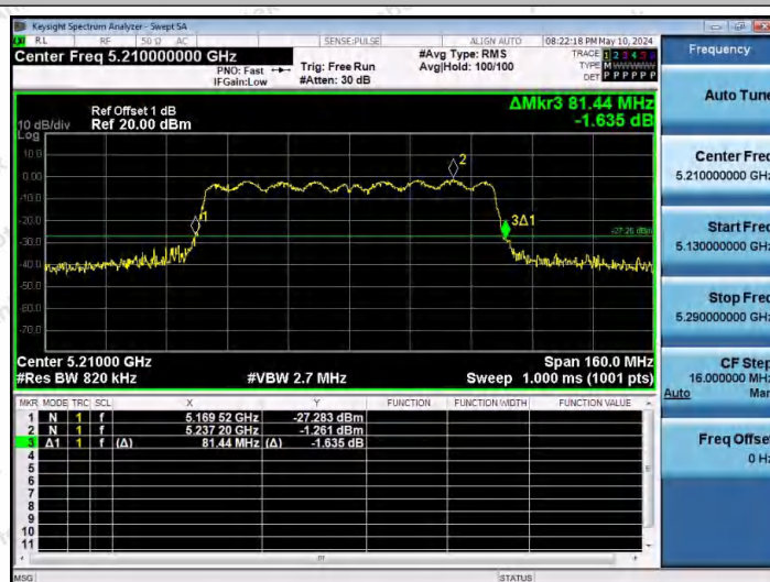
11AC80SISO-Ant1-5210
