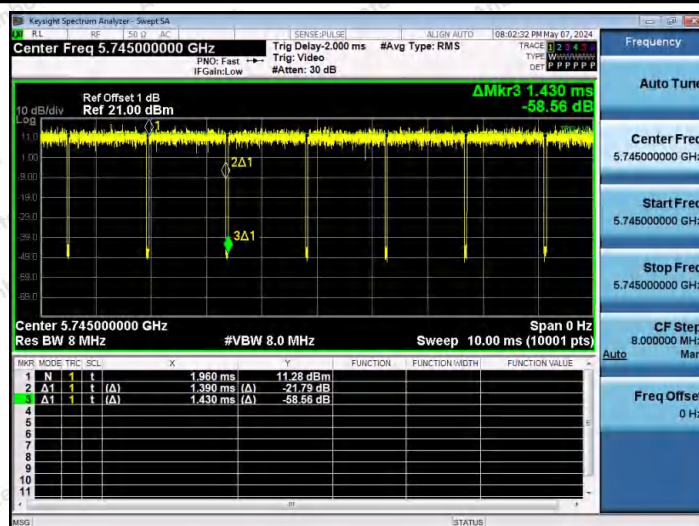
NTNV-11A-Ant1-5745
