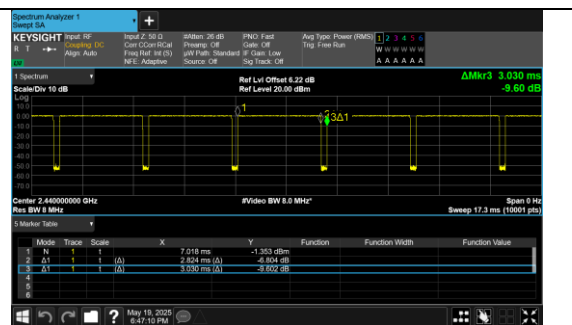
BLE 1M_Channel 19
