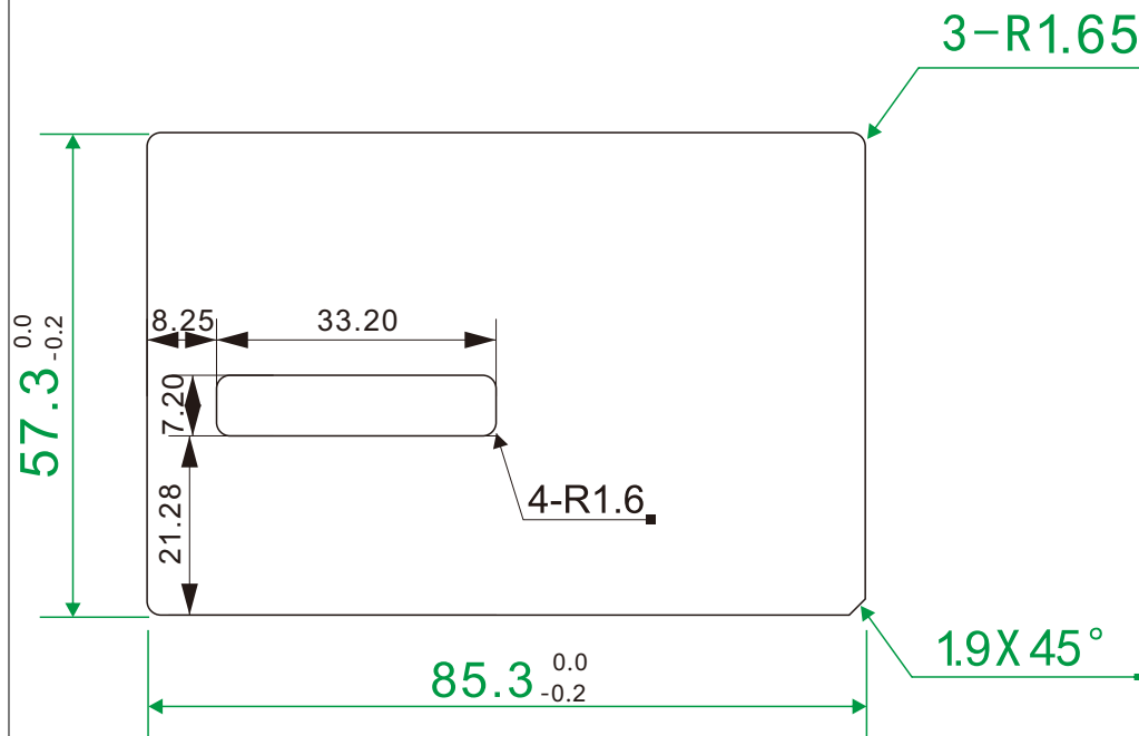
(尺寸图)
