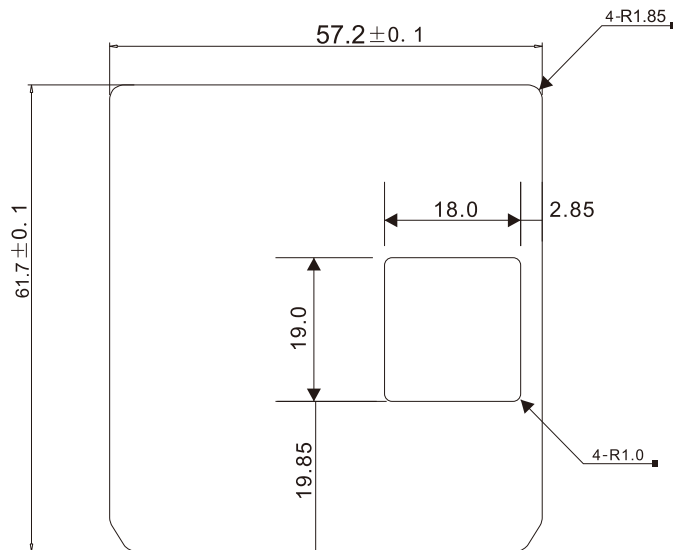
尺寸图
