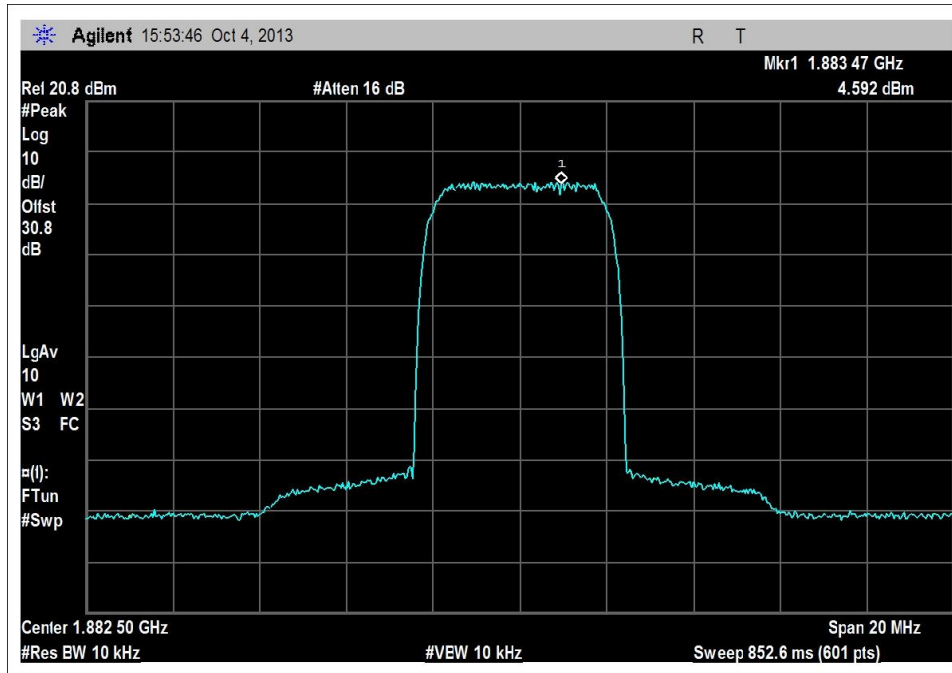
1850 - 1910MHz UL, WCDMA - Input
