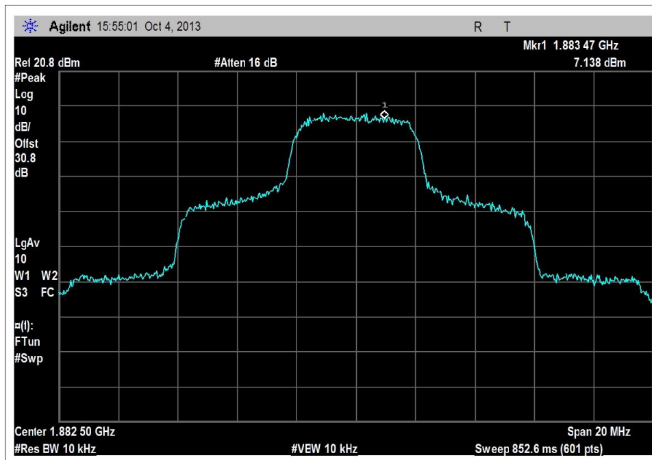
1850 - 1910MHz UL, WCDMA - Output
