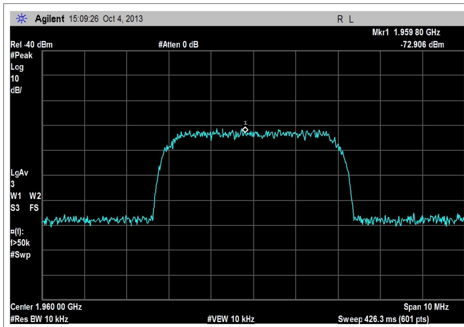
1930 - 1990MHz DL, WCDMA - Output
