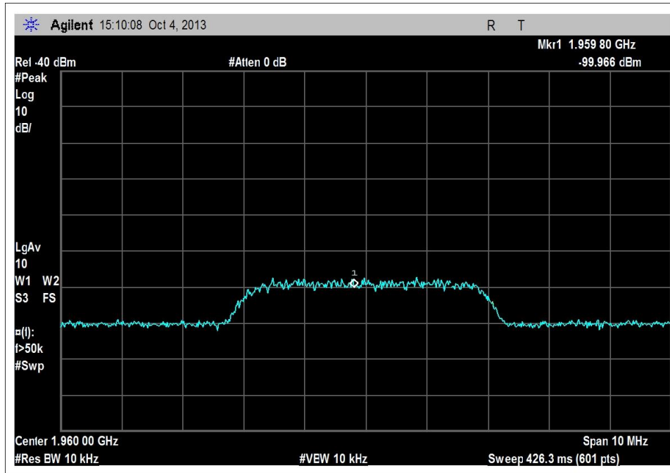
1930 - 1990MHz DL, WCDMA - Input
