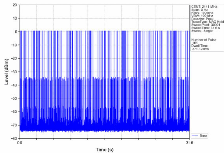
Pi/4DQPSK_2DH3_HOPP_Ant1_NTNV
