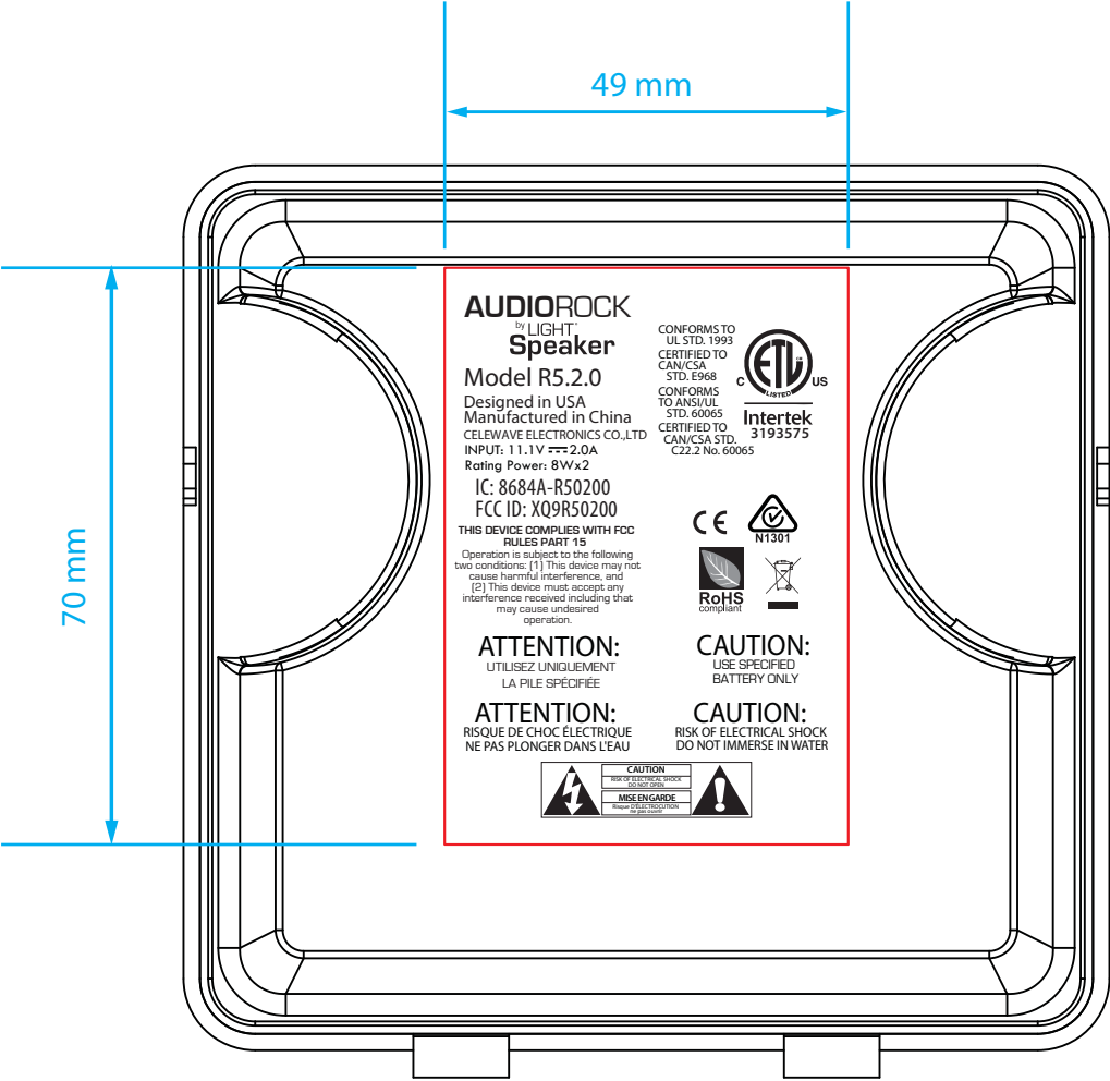
Label Dimensions
