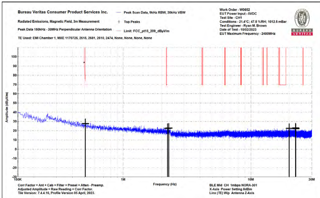
0.15-30MHz Perpendicular
