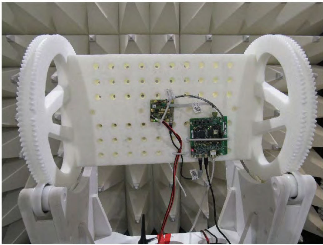
EUT Test Setup
