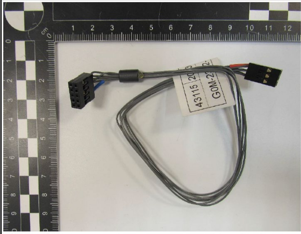
SPI Cable
