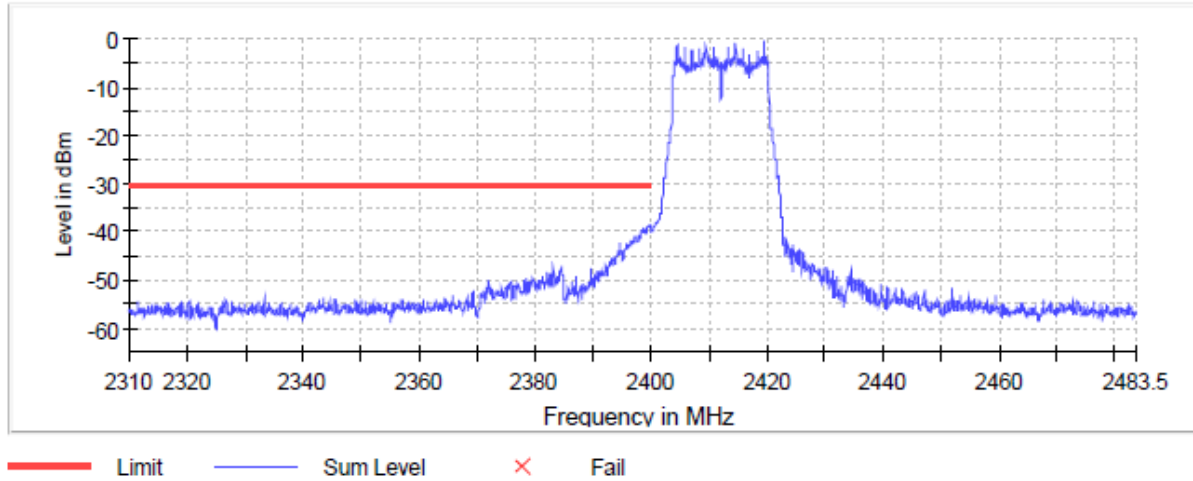
Band Edge
