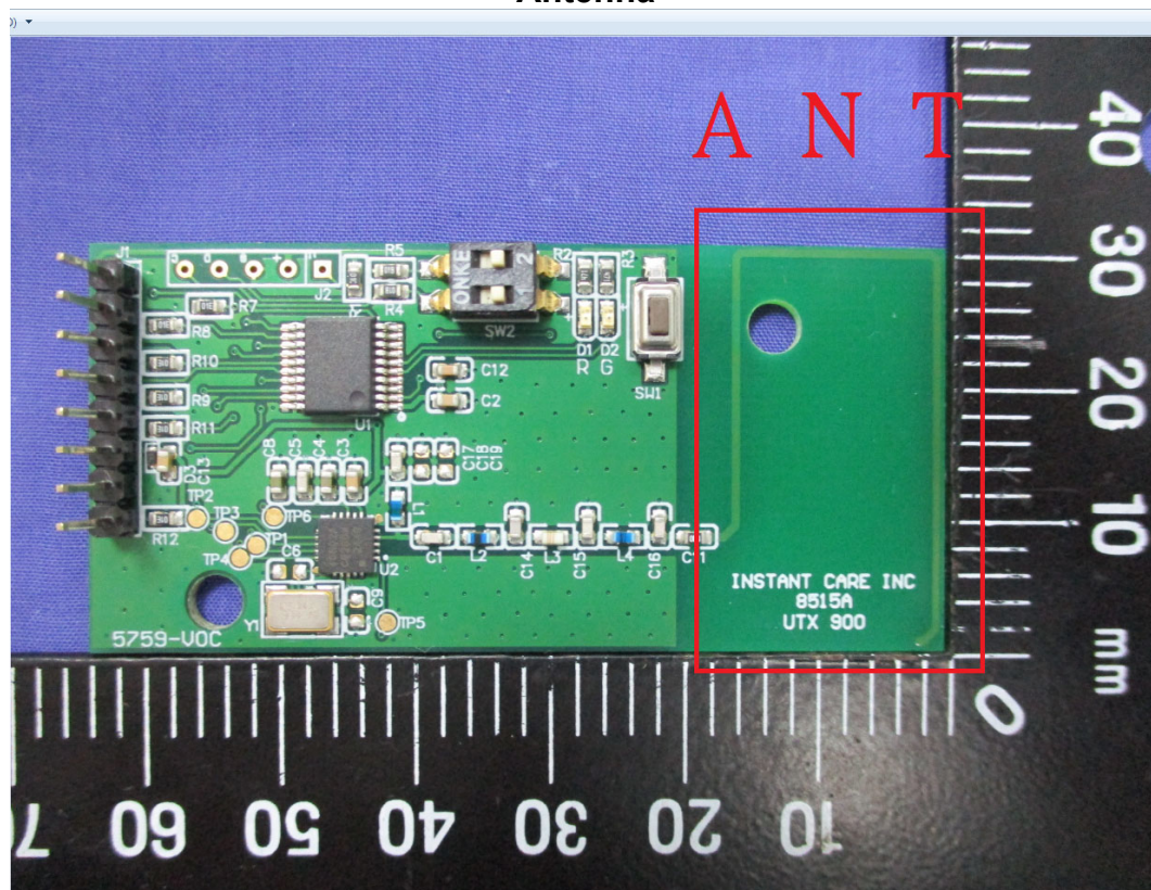
Antenna
