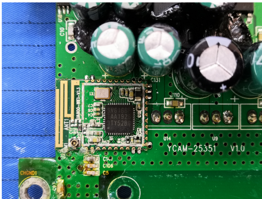
Wi-Fi Module
