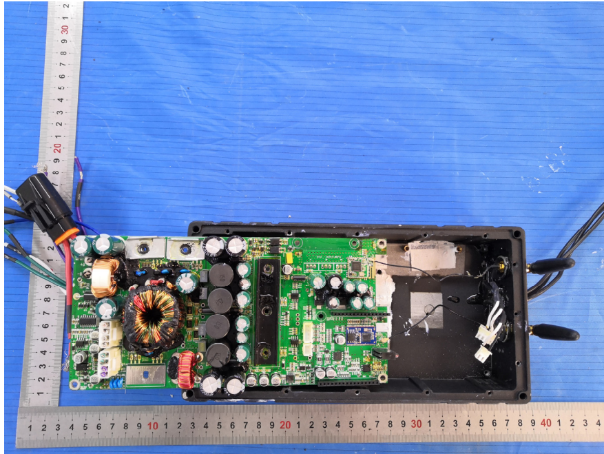
Wi-Fi Module
