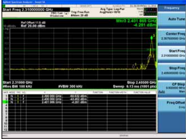
2402MHz(2.3GHz – 2.4GHz)
