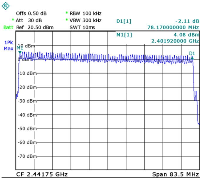
Modulation: \pi/4 DQPSK
