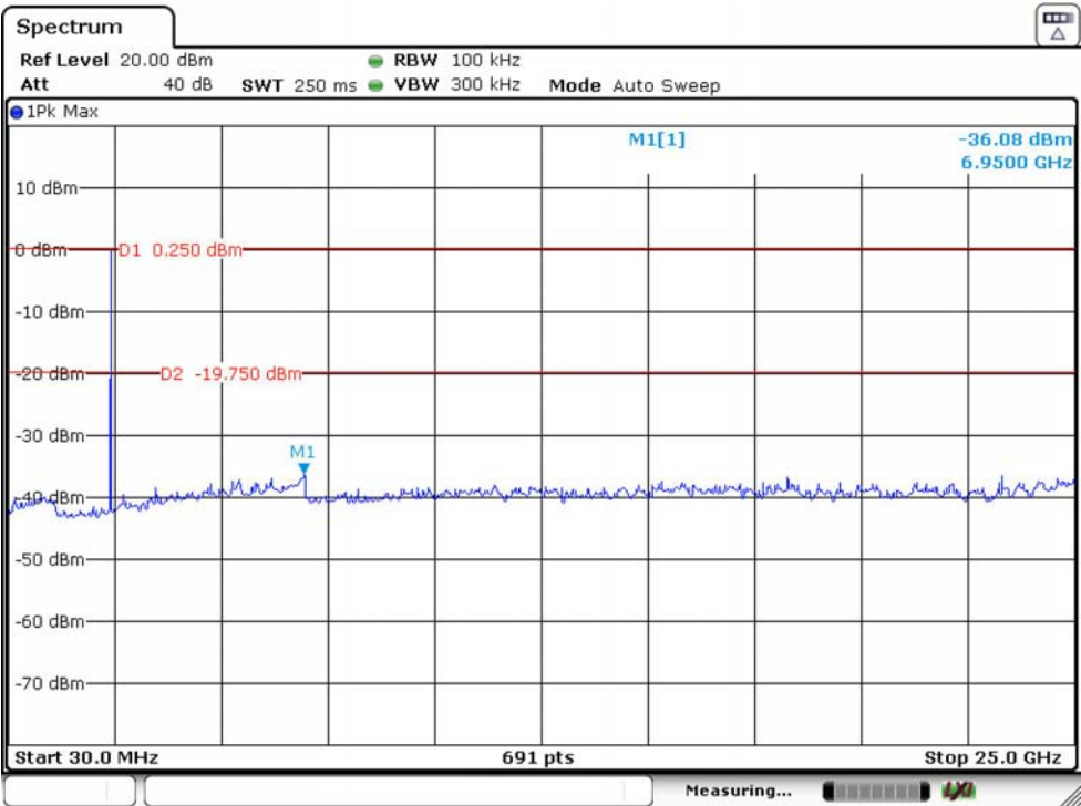
GFSK 2441 MHz ANT A1
