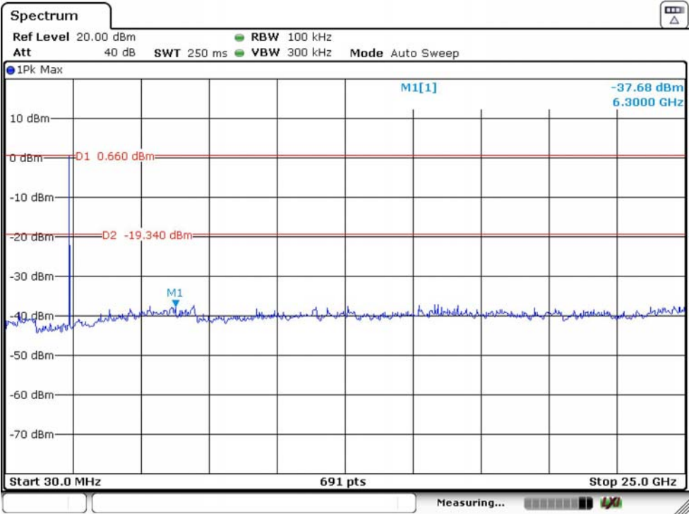
GFSK 2404 MHz ANT A1
