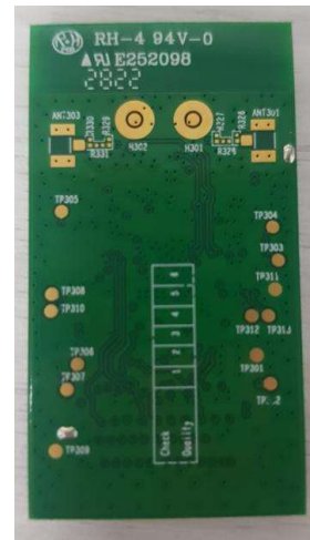
Fig 5.2 5G_MODULE_FPC Module
