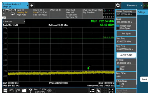
BLE_2M-Ant1-2440-30~1000-PASS
