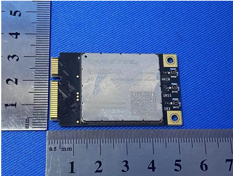
Type: MINIPCIE
