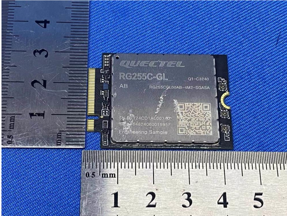
Type: M.2
