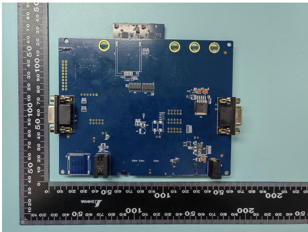
EG915Q-AF + EVB_Bottom
