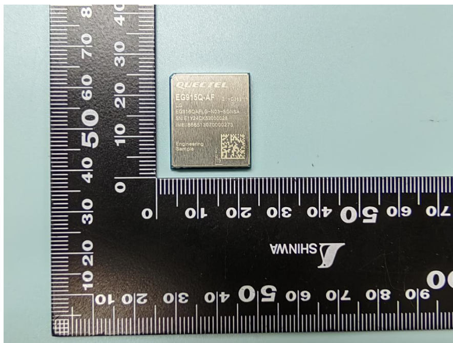
EG915Q-AF_Top
