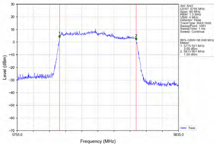
802.11ax(HE40) HCH 5795MHz RU484 Left Ant2 NTN
