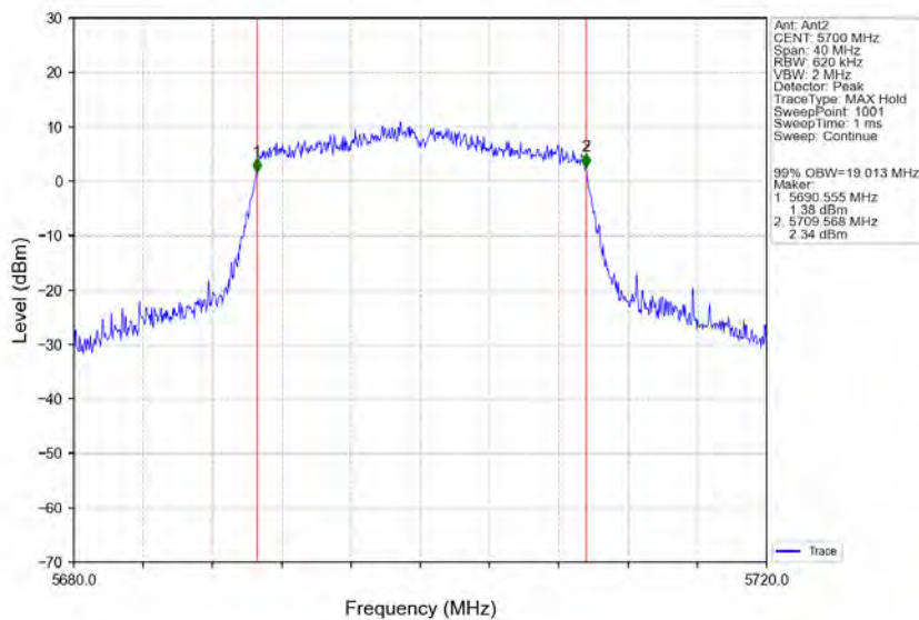
802.11ax(HE20) HCH 5700MHz RU242 Left Ant2 NTN
