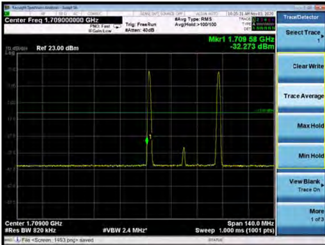
CA-4C-12A 64QAM 20MHz+20MHz+20MHz CH-Low, 100%RB
