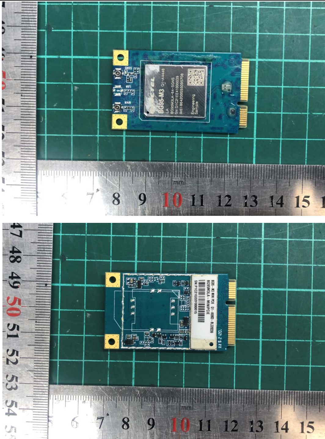
BG95-M3 MINIPCIE
