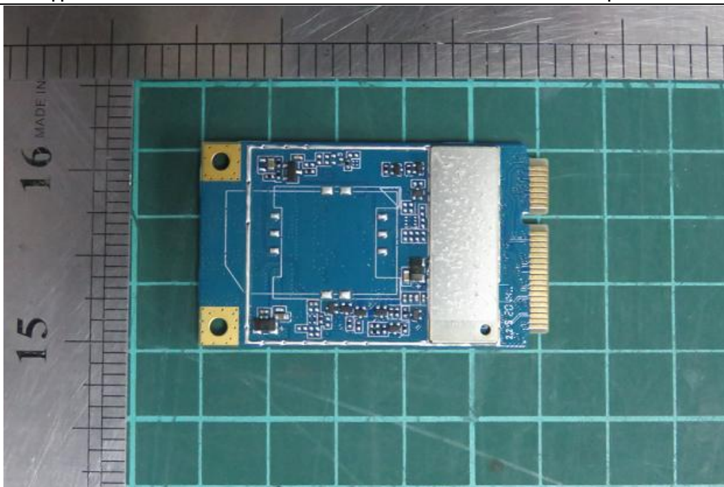
BG95-M3 MINIPCIE
