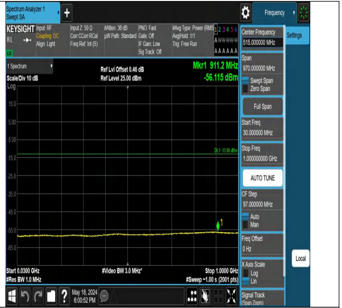
Band2-9538-2-30~1000MHz-PASS
