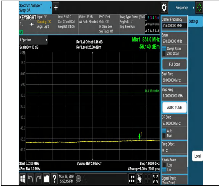
Band2-9538-1-30~1000MHz-PASS
