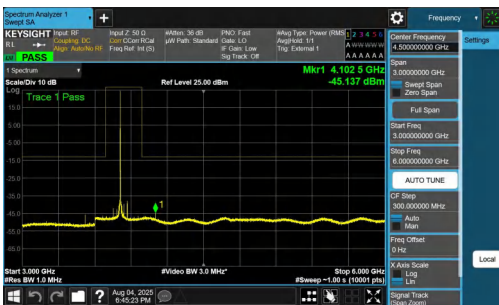
NTNV-n77(3700-3980)-PC2-30-60-M-DFT-QPSK-Inner_1RB_Left-3000-6000-PASS
