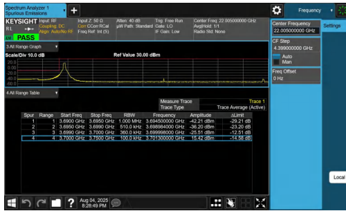
NTNV-n77(3700-3980)-PC2-30-50-L-DFT-QPSK-Edge_1RB_Left-PASS
