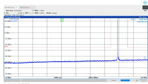
NTNV-n41-PC2-30-25-M-DFT-QPSK-Inner_1RB_Left-1000-3000-PASS
