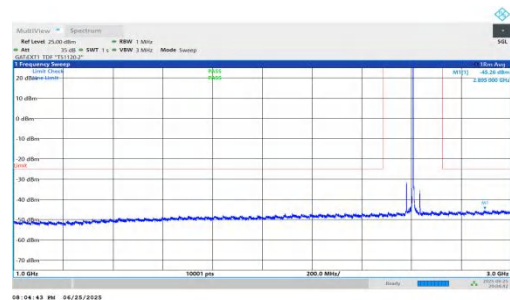
NTNV-n41-PC2-30-30-M-DFT-QPSK-Inner_1RB_Right-1000-3000- -PASS
