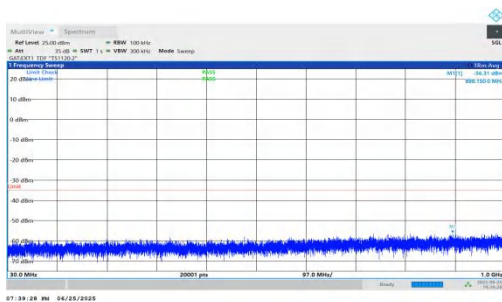
NTNV-n41-PC2-30-25-L-DFT-QPSK-Inner_1RB_Left-30-1000-PASS
