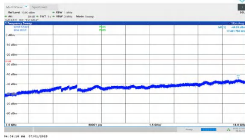
NTVN-n41-PC2-30-20-L-DFT-QPSK-Inner_1RB_Left-3000-18000 -PASS
