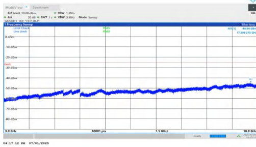
NTVN-n41-PC2-30-30-L-DFT-QPSK-Inner_1RB_Left-3000-18000 -PASS
