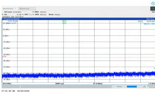
NTNV-n41-PC2-30-20-L-DFT-QPSK-Inner_1RB_Left-30-1000-PASS
