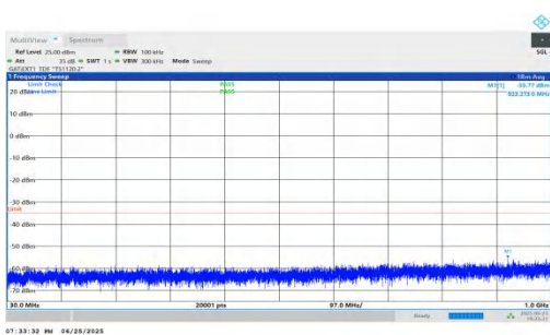
NTVN-n41-PC2-30-20-H-DFT-QPSK-Inner_1RB_Left-30-1000-P ASS
