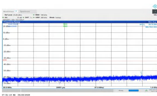
NTVN-n41-PC2-30-25-H-DFT-QPSK-Inner_1RB_Left-30-1000-P ASS
