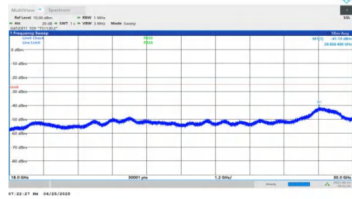
NTVN-n41-PC2-30-20-L-DFT-QPSK-Inner_1RB_Left-18000-3000 0-PASS
