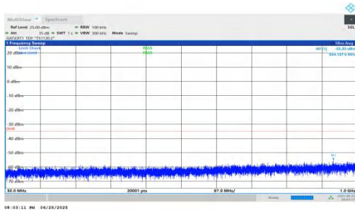
NTNV-n41-PC2-30-30-M-DFT-QPSK-Inner_1RB_Left-30-1000-PASS
