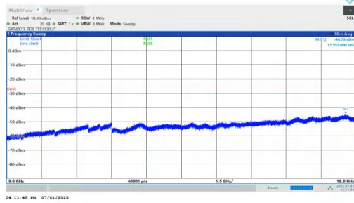
NTVN-n41-PC2-30-25-L-DFT-QPSK-Inner_1RB_Left-3000-18000 -PASS
