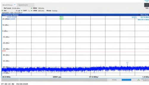
NTNV-n38-PC3-30-20-M-DFT-QPSK-Inner_1RB_Left-30-1000-PASS
