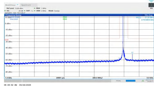
NTNV-n38-PC3-30-25-M-DFT-QPSK-Inner_1RB_Left-1000-3000-PASS
