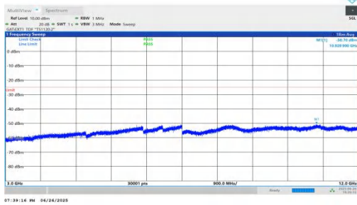
NTNV-n38-PC3-30-20-L-DFT-QPSK-Inner_1RB_Left-3000-12000 -PASS
