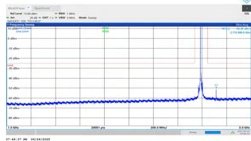
NTNV-n38-PC3-30-20-M-DFT-QPSK-Inner_1RB_Left-1000-3000-PASS
