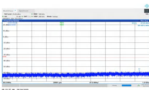
NTNV-n38-PC3-30-25-H-DFT-QPSK-Inner_1RB_Left-30-1000-P ASS
