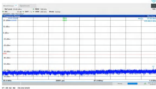
NTNV-n38-PC3-30-20-L-DFT-QPSK-Inner_1RB_Left-30-1000-PASS
