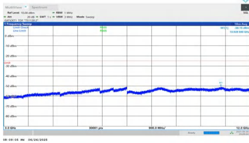
NTNV-n38-PC3-30-25-M-DFT-QPSK-Inner_1RB_Left-3000-1200 0-PASS
