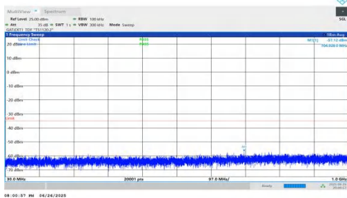
NTNV-n38-PC3-30-25-L-DFT-QPSK-Inner_1RB_Left-30-1000-PA SS
