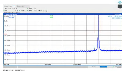
NTNV-n38-PC3-30-20-M-DFT-QPSK-Inner_1RB_Right-1000-3000- -PASS
