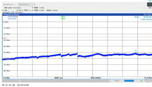
NTNV-n38-PC3-30-25-L-DFT-QPSK-Inner_1RB_Left-3000-12000 -PASS
