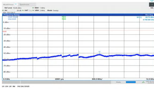
NTVN-n25-PC3-15-10-L-DFT-QPSK-Inner_1RB_Left-3000-12000 -PASS
