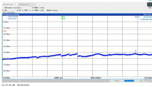
NTNV-n25-PC3-15-15-L-DFT-QPSK-Inner_1RB_Left-3000-12000 -PASS
