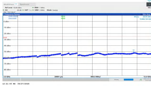
NTNV-n7-PC3-15-20-M-DFT-QPSK-Inner_1RB_Left-3000-12000 -PASS
