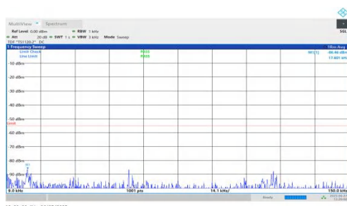
NTVN-n7-PC3-15-20-M-DFT-BPSK-Inner_1RB_Right-0.009-0.15 -PASS
