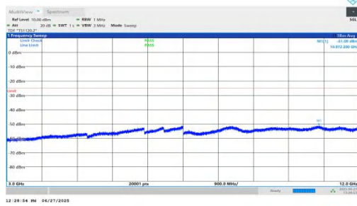
NTNV-n7-PC3-15-25-M-DFT-QPSK-Inner_1RB_Left-3000-12000 -PASS
