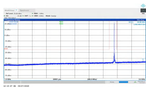
NTNV-n7-PC3-15-15-H-DFT-QPSK-Inner_1RB_Left-1000-3000-P ASS
