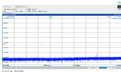
NTNV-n7-PC3-15-30-L-DFT-QPSK-Inner_1RB_Left-30-1000-PA SS
