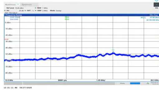
NTNV-n7-PC3-15-20-M-DFT-QPSK-Inner_1RB_Left-12000-26500 -PASS
