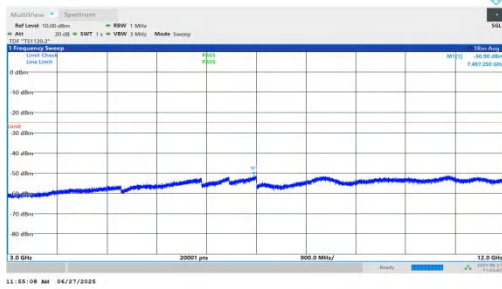
NTNV-n7-PC3-15-5-L-DFT-QPSK-Inner_1RB_Left-3000-12000-P ASS
