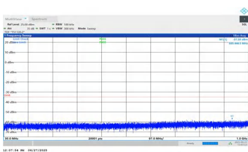
NTNV-n7-PC3-15-10-H-DFT-QPSK-Inner_1RB_Left-30-1000-P ASS
