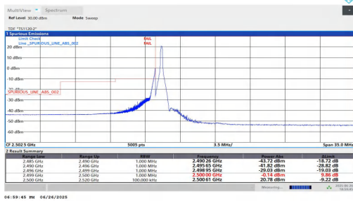
NTNV-n7-PC3-15-40-L-DFT-BPSK-Edge_1RB_Left
