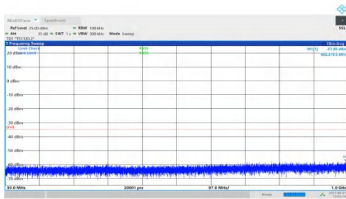
NTNV-n7-PC3-15-10-M-DFT-QPSK-Inner_1RB_Left-30-1000-PASS
