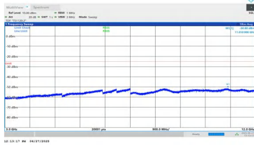
NTNV-n7-PC3-15-15-M-DFT-QPSK-Inner_1RB_Left-3000-12000 -PASS
