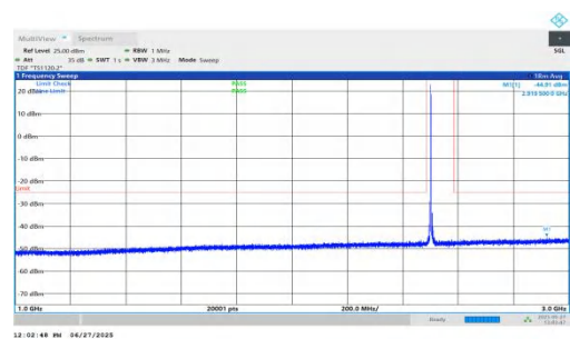
NTVN-n7-PC3-15-10-L-DFT-QPSK-Inner_1RB_Left-1000-3000-PA SS
