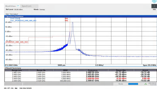
NTNV-n7-PC3-15-40-L-DFT-QPSK-Edge_1RB_Left
