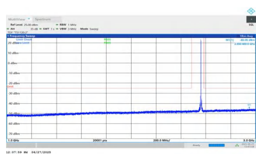
NTNV-n7-PC3-15-10-H-DFT-QPSK-Inner_1RB_Left-1000-3000-P ASS
