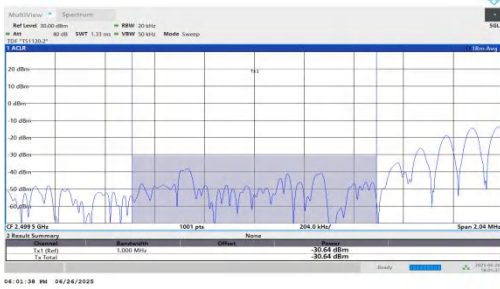
NTNV-n7-PC3-15-50-L-DFT-QPSK-Edge_1RB_Left-PASS
