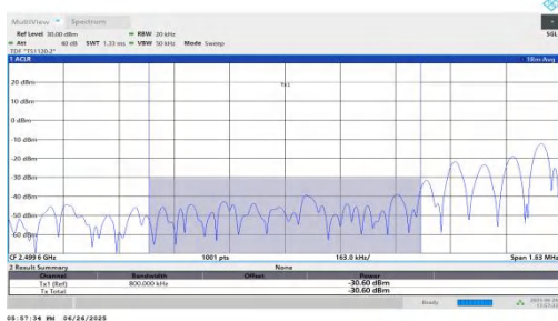
NTNV-n7-PC3-15-40-L-DFT-QPSK-Edge_1RB_Left-PASS
