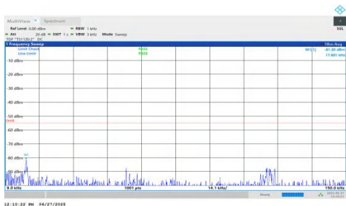
NTNV-n7-PC3-15-15-L-DFT-QPSK-Inner_1RB_Left-0.009-0.15-P ASS
