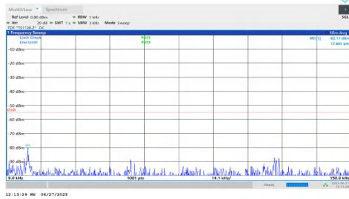
NTNV-n7-PC3-15-15-M-DFT-QPSK-Inner_1RB_Right-0.009-0.15 -PASS
