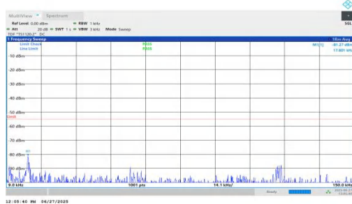
NTNV-n7-PC3-15-10-M-DFT-QPSK-Inner_1RB_Right-0.009-0.15 -PASS
