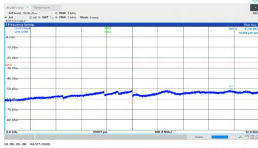
NTNV-n7-PC3-15-10-M-DFT-QPSK-Inner_1RB_Left-3000-12000 -PASS
