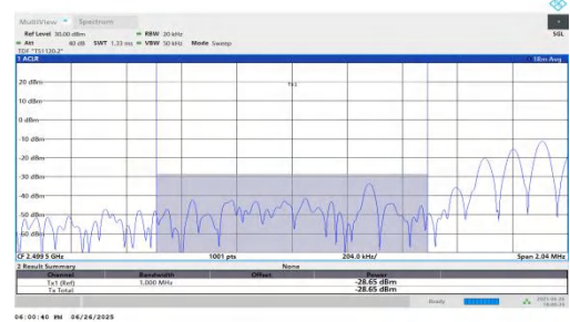
NTNV-n7-PC3-15-50-L-DFT-BPSK-Edge_1RB_Left-PASS
