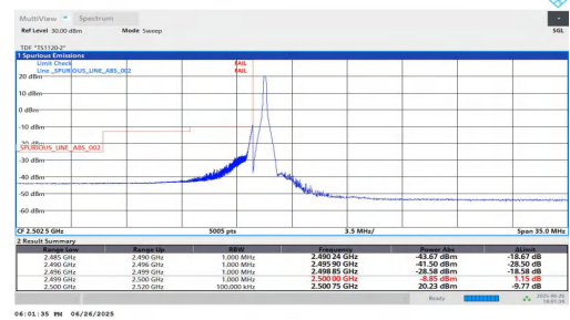
NTNV-n7-PC3-15-50-L-DFT-QPSK-Edge_1RB_Left
