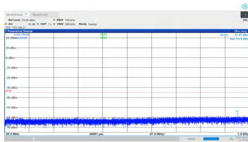
NTNV-n7-PC3-15-15-M-DFT-QPSK-Inner_1RB_Left-30-1000-PASS
