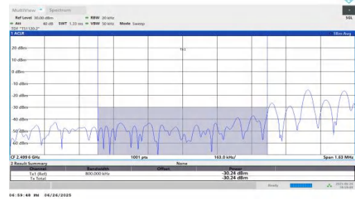
NTNV-n7-PC3-15-40-L-DFT-BPSK-Edge_1RB_Left-PASS
