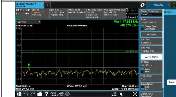
42-42-20MHz-20MHz-QPSK-QPSK-42190-42388-1RB#99-0RB# 0-0.009~0.15MHz-PASS
