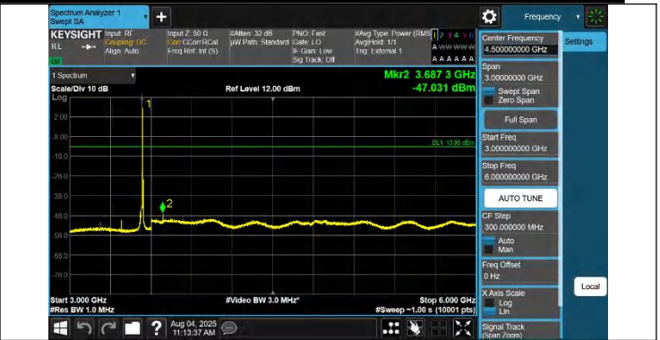
42-42-20MHz-15MHz-QPSK-QPSK-42841-43012-1RB#99-0RB# 0-3000~6000MHz-PASS
