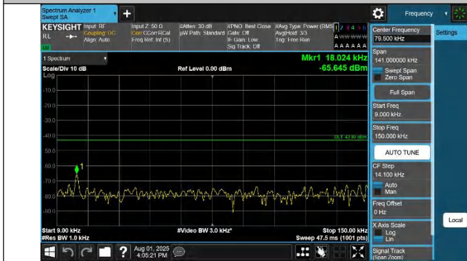
42-42-20MHz-20MHz-QPSK-QPSK-42792-42990-1RB#99-0RB# 0-0.009~0.15MHz-PASS
