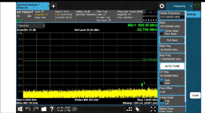
42-42-20MHz-20MHz-QPSK-QPSK-42491-42689-1RB#99-0RB# 0-30~1000MHz-PASS
