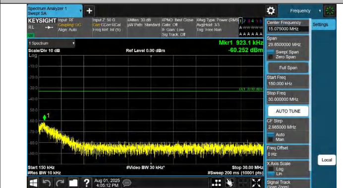
42-42-20MHz-20MHz-QPSK-QPSK-42792-42990-1RB#0-0RB#0- 0.15~30MHz-PASS
