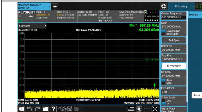
42-42-20MHz-20MHz-QPSK-QPSK-42792-42990-1RB#99-0RB# 0-30~1000MHz-PASS
