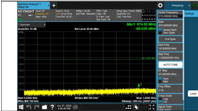
66-66-20MHz-10MHz-QPSK-QPSK-132473-132617-1RB#0-1RB #49-30~1000MHz-PASS
