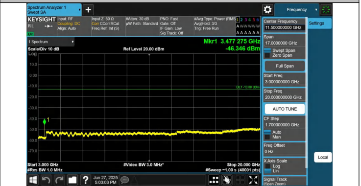
66-66-20MHz-15MHz-QPSK-QPSK-132348-132519-1RB#0-0RB #0-3000~20000MHz-PASS
