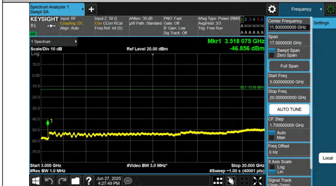
66-66-20MHz-10MHz-QPSK-QPSK-132373-132517-1RB#99-0R B#0-3000~20000MHz-PASS
