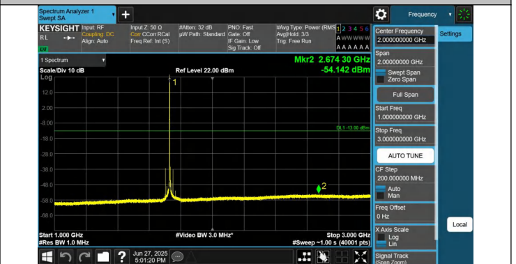
66-66-20MHz-15MHz-QPSK-QPSK-132072-132243-1RB#99-0R B#0-1000~3000MHz-PASS
