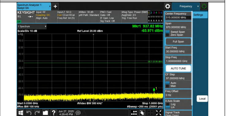
66-66-20MHz-10MHz-QPSK-QPSK-132473-132617-1RB#99-0R B#0-30~1000MHz-PASS
