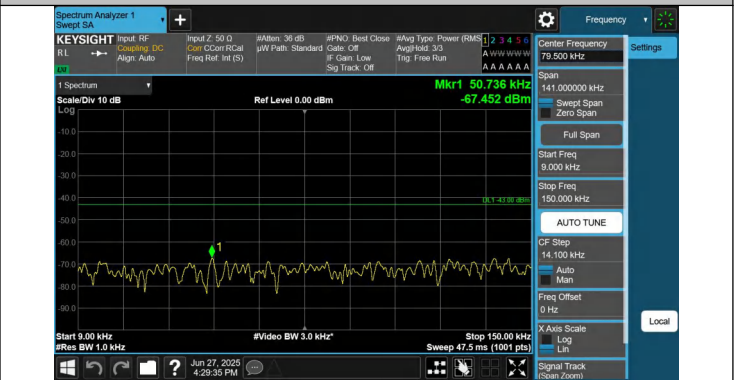
66-66-20MHz-10MHz-QPSK-QPSK-132473-132617-1RB#99-0R B#0-0.009~0.15MHz-PASS
