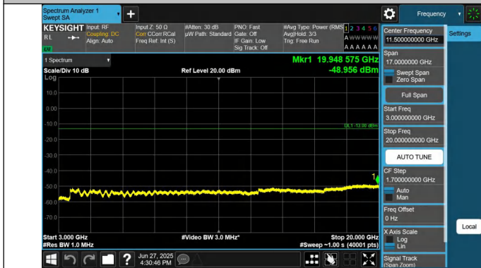
66-66-20MHz-10MHz-QPSK-QPSK-132473-132617-1RB#0-1RB #49-3000~20000MHz-PASS
