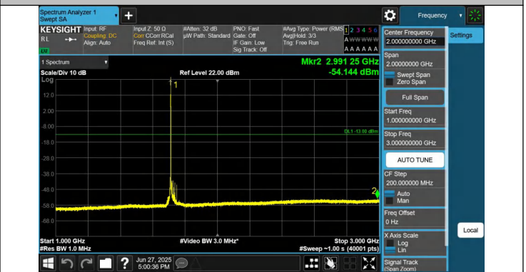
66-66-20MHz-15MHz-QPSK-QPSK-132072-132243-1RB#0-0RB #0-1000~3000MHz-PASS
