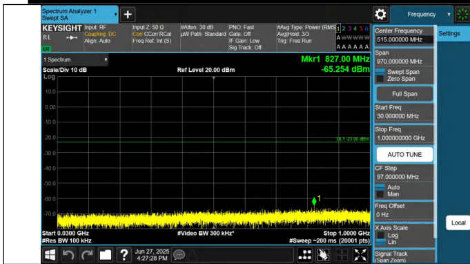
66-66-20MHz-10MHz-QPSK-QPSK-132373-132517-1RB#99-0R B#0-30~1000MHz-PASS
