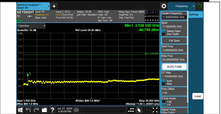
66-66-20MHz-10MHz-QPSK-QPSK-132473-132617-1RB#99-0R B#0-3000~20000MHz-PASS
