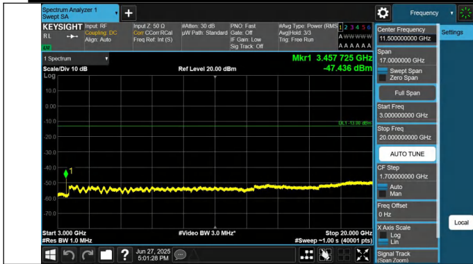
66-66-20MHz-15MHz-QPSK-QPSK-132072-132243-1RB#99-0R B#0-3000~20000MHz-PASS
