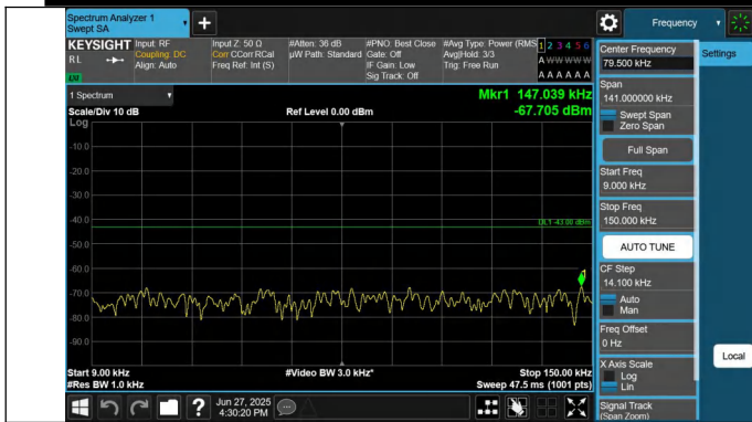
66-66-20MHz-10MHz-QPSK-QPSK-132473-132617-1RB#0-1RB #49-0.009~0.15MHz-PASS
