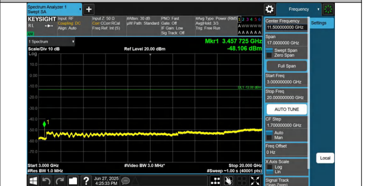
66-66-20MHz-10MHz-QPSK-QPSK-132072-132216-1RB#99-0R B#0-3000~20000MHz-PASS
