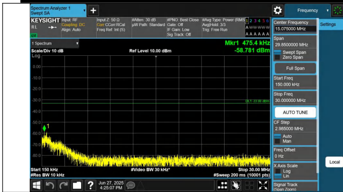
66-66-20MHz-10MHz-QPSK-QPSK-132072-132216-1RB#99-0R B#0-0.15~30MHz-PASS
