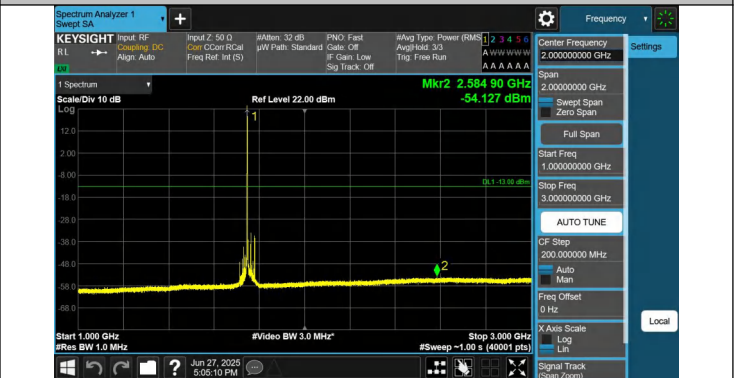
66-66-20MHz-15MHz-QPSK-QPSK-132423-132594-1RB#0-0RB #0-1000~3000MHz-PASS
