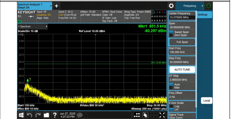
66-66-20MHz-10MHz-QPSK-QPSK-132373-132517-1RB#99-0R B#0-0.15~30MHz-PASS
