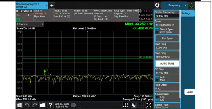
66-66-20MHz-10MHz-QPSK-QPSK-132373-132517-1RB#0-1RB #49-0.009~0.15MHz-PASS
