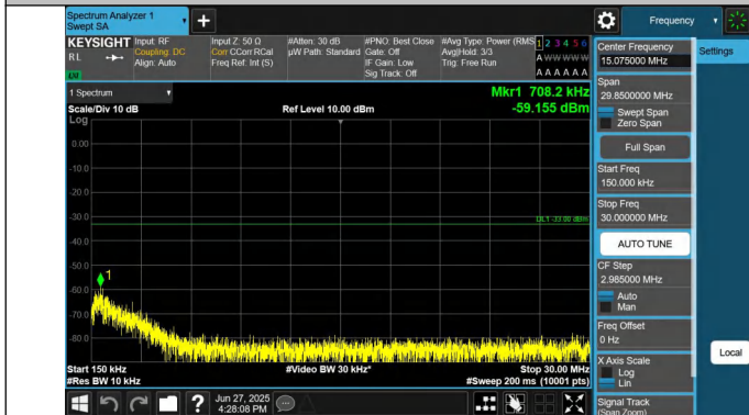
66-66-20MHz-10MHz-QPSK-QPSK-132373-132517-1RB#0-1RB #49-0.15~30MHz-PASS
