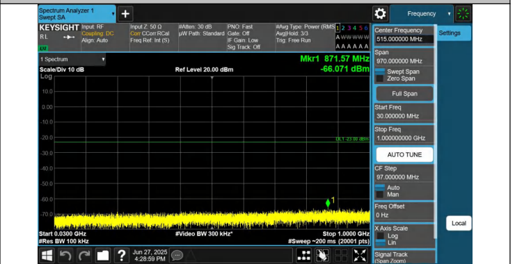
66-66-20MHz-10MHz-QPSK-QPSK-132473-132617-1RB#0-0RB #0-30~1000MHz-PASS
