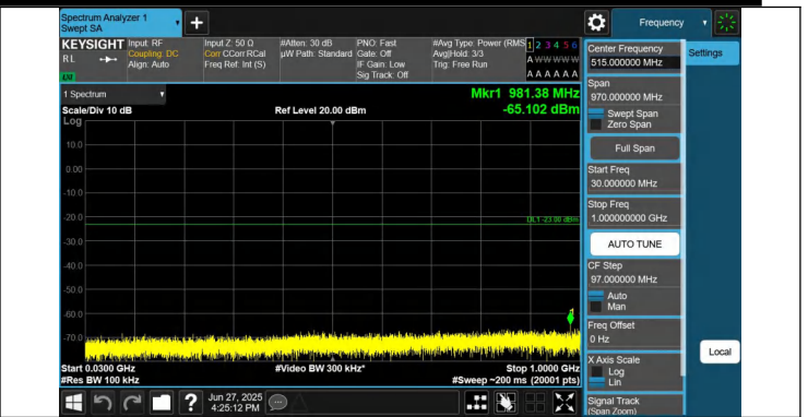
66-66-20MHz-10MHz-QPSK-QPSK-132072-132216-1RB#99-0R B#0-30~1000MHz-PASS
