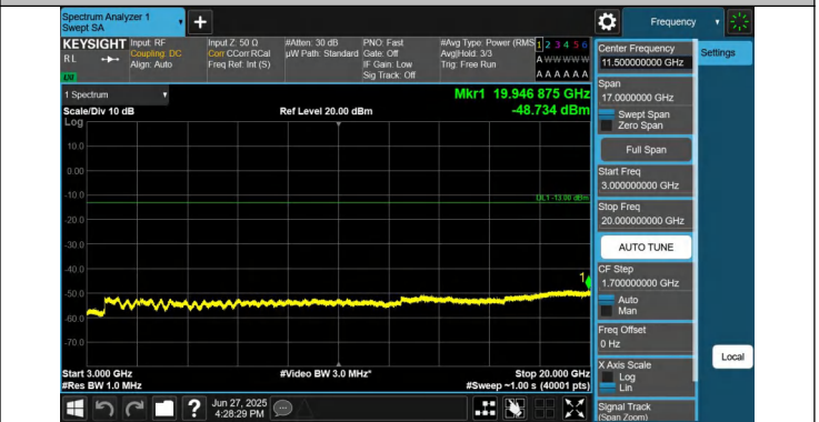
66-66-20MHz-10MHz-QPSK-QPSK-132373-132517-1RB#0-1RB #49-3000~20000MHz-PASS
