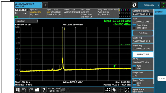
66-66-20MHz-10MHz-QPSK-QPSK-132473-132617-1RB#99-0R B#0-1000~3000MHz-PASS
