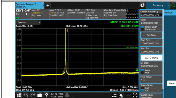
66-66-20MHz-10MHz-QPSK-QPSK-132473-132617-1RB#0-0RB #0-1000~3000MHz-PASS
