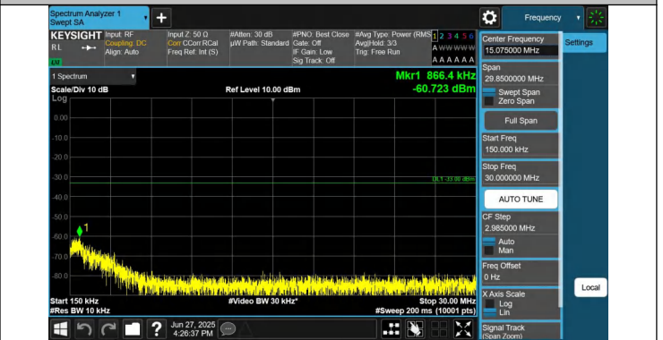
66-66-20MHz-10MHz-QPSK-QPSK-132373-132517-1RB#0-0RB #0-0.15~30MHz-PASS
