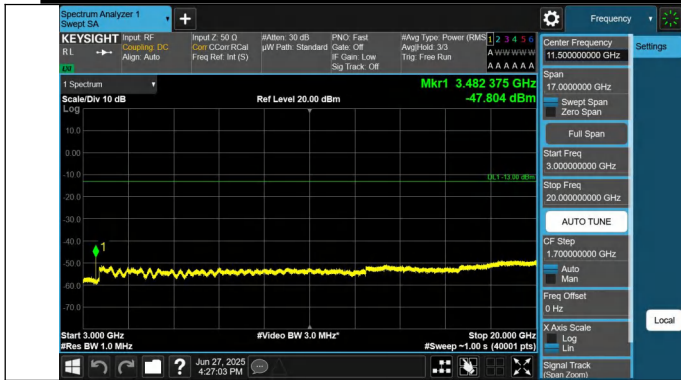
66-66-20MHz-10MHz-QPSK-QPSK-132373-132517-1RB#0-0RB #0-3000~20000MHz-PASS
