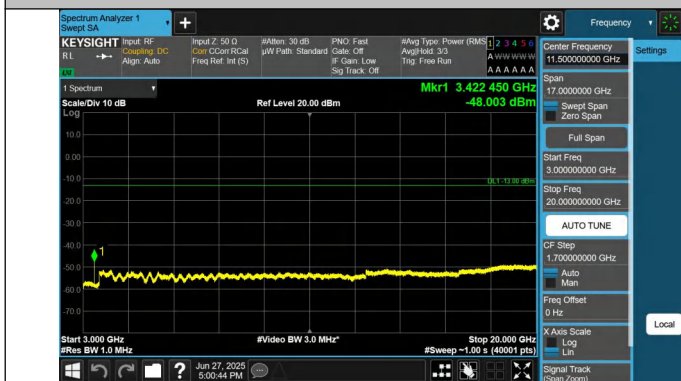
66-66-20MHz-15MHz-QPSK-QPSK-132072-132243-1RB#0-0RB #0-3000~20000MHz-PASS
