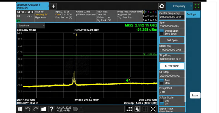
66-66-20MHz-10MHz-QPSK-QPSK-132373-132517-1RB#99-0R B#0-1000~3000MHz-PASS
