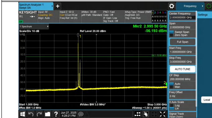
66-66-20MHz-10MHz-QPSK-QPSK-132373-132517-1RB#0-1RB #49-1000~3000MHz-PASS
