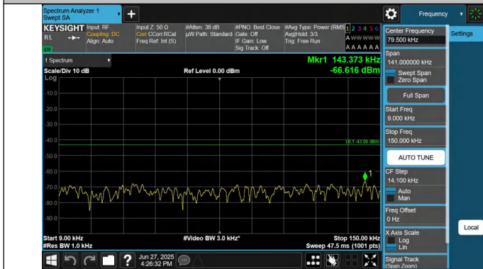
66-66-20MHz-10MHz-QPSK-QPSK-132373-132517-1RB#0-0RB #0-0.009~0.15MHz-PASS
