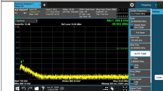
66-66-20MHz-10MHz-QPSK-QPSK-132473-132617-1RB#99-0R B#0-0.15~30MHz-PASS
