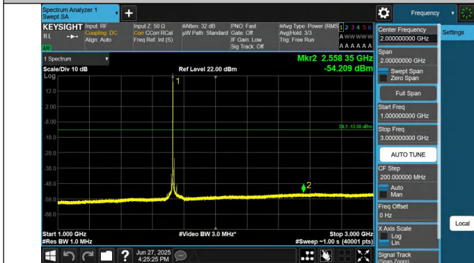
66-66-20MHz-10MHz-QPSK-QPSK-132072-132216-1RB#99-0R B#0-1000~3000MHz-PASS
