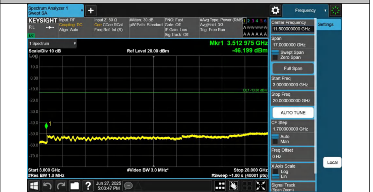
66-66-20MHz-15MHz-QPSK-QPSK-132348-132519-1RB#99-0R B#0-3000~20000MHz-PASS
