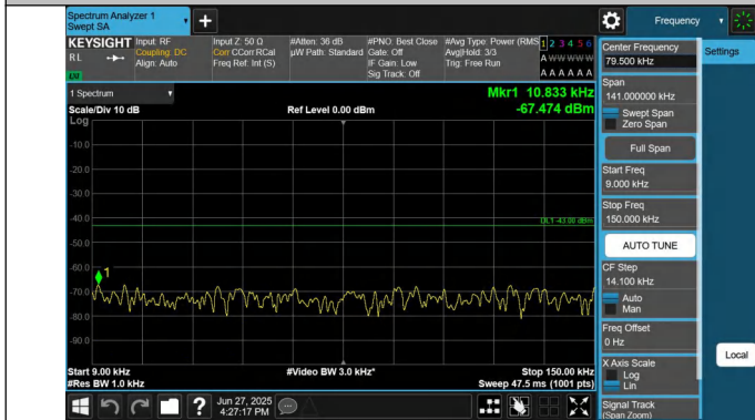
66-66-20MHz-10MHz-QPSK-QPSK-132373-132517-1RB#99-0R B#0-0.009~0.15MHz-PASS
