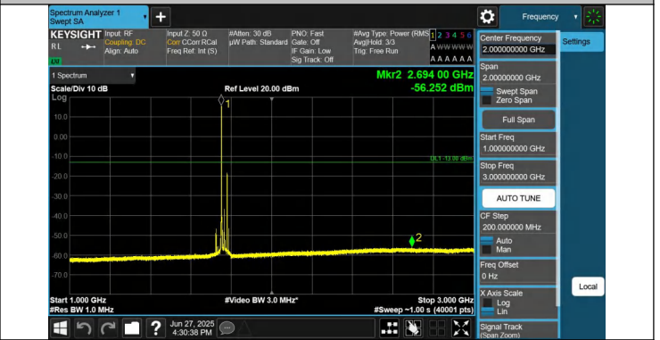
66-66-20MHz-10MHz-QPSK-QPSK-132473-132617-1RB#0-1RB #49-1000~3000MHz-PASS
