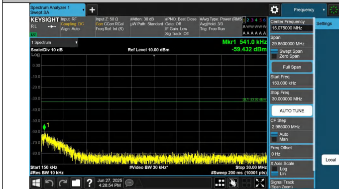
66-66-20MHz-10MHz-QPSK-QPSK-132473-132617-1RB#0-0RB #0-0.15~30MHz-PASS
