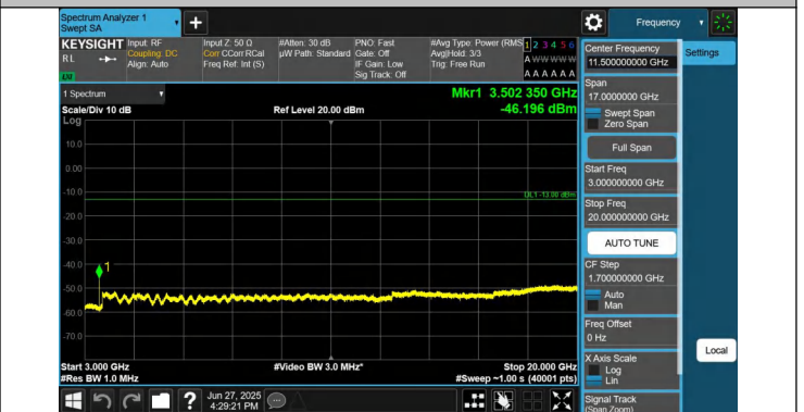
66-66-20MHz-10MHz-QPSK-QPSK-132473-132617-1RB#0-0RB #0-3000~20000MHz-PASS
