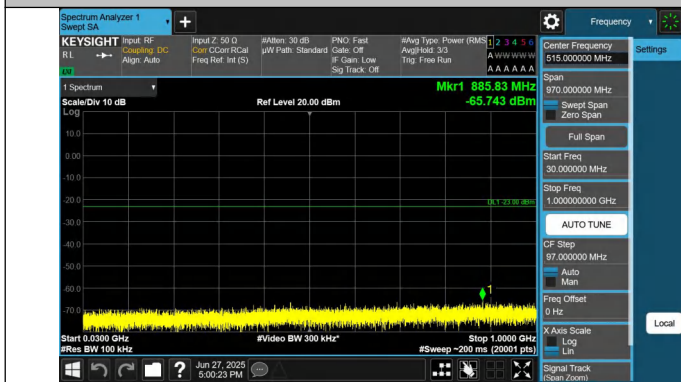
66-66-20MHz-15MHz-QPSK-QPSK-132072-132243-1RB#0-0RB #0-30~1000MHz-PASS
