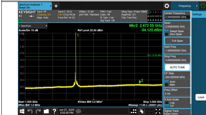
66-66-20MHz-15MHz-QPSK-QPSK-132348-132519-1RB#0-0RB #0-1000~3000MHz-PASS
