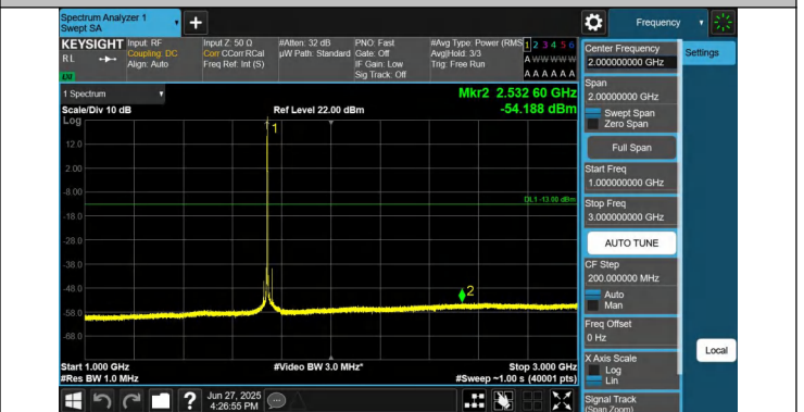
66-66-20MHz-10MHz-QPSK-QPSK-132373-132517-1RB#0-0RB #0-1000~3000MHz-PASS
