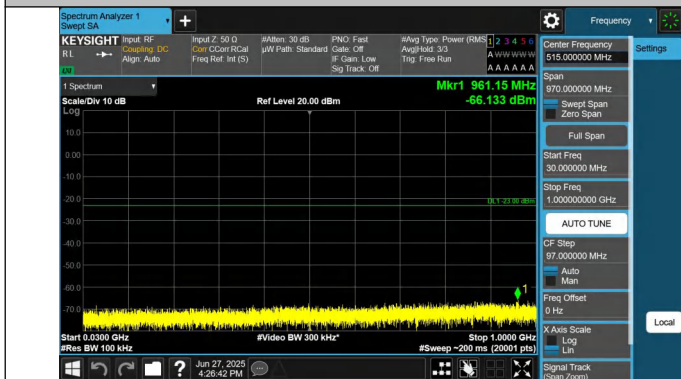
66-66-20MHz-10MHz-QPSK-QPSK-132373-132517-1RB#0-0RB #0-30~1000MHz-PASS
