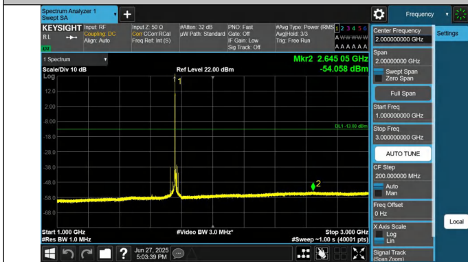
66-66-20MHz-15MHz-QPSK-QPSK-132348-132519-1RB#99-0R B#0-1000~3000MHz-PASS
