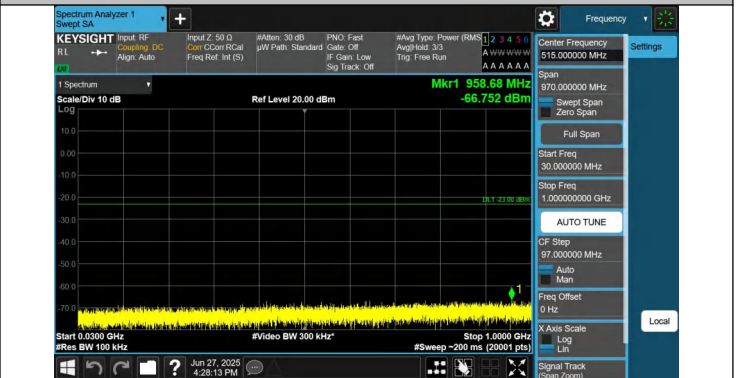
66-66-20MHz-10MHz-QPSK-QPSK-132373-132517-1RB#0-1RB #49-30~1000MHz-PASS
