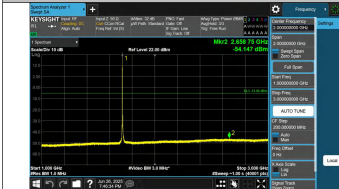
66-66-5MHz-20MHz-QPSK-QPSK-132027-132171-1RB#0-1RB# 99-1000~3000MHz-PASS
