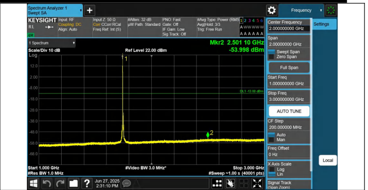
66-66-10MHz-15MHz-QPSK-QPSK-132351-132471-1RB#0-0RB #0-1000~3000MHz-PASS
