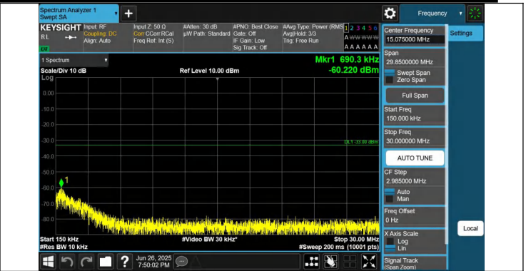
66-66-5MHz-20MHz-QPSK-QPSK-132428-132572-1RB#0-0RB# 0-0.15~30MHz-PASS
