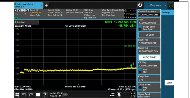
66-66-5MHz-20MHz-QPSK-QPSK-132428-132572-1RB#0-1RB# 99-3000~20000MHz-PASS
