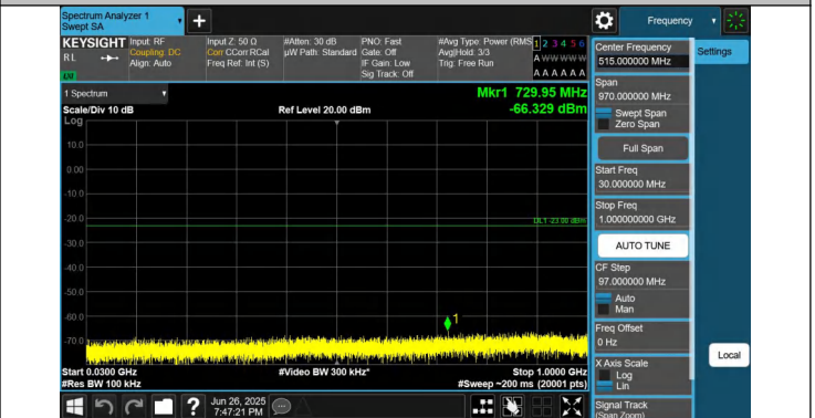
66-66-5MHz-20MHz-QPSK-QPSK-132328-132472-1RB#0-0RB# 0-30~1000MHz-PASS
