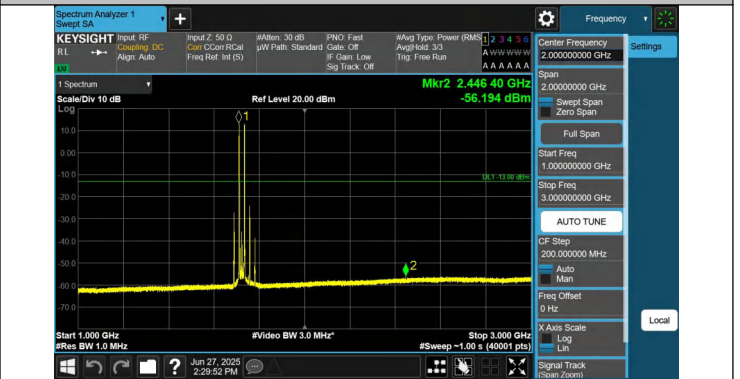
66-66-10MHz-15MHz-QPSK-QPSK-132025-132145-1RB#0-1RB #74-1000~3000MHz-PASS
