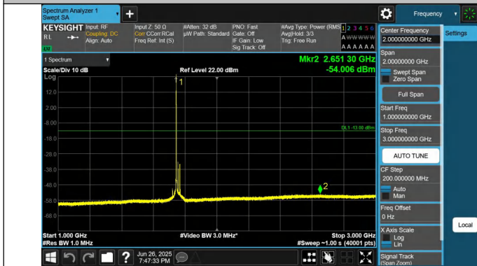
66-66-5MHz-20MHz-QPSK-QPSK-132328-132472-1RB#0-0RB# 0-1000~3000MHz-PASS
