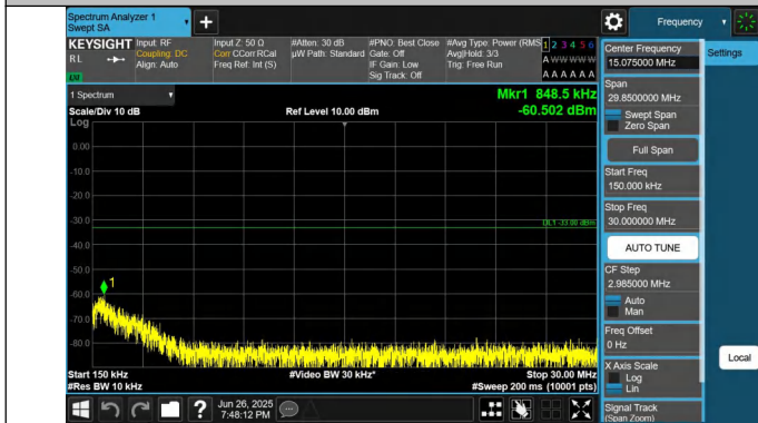
66-66-5MHz-20MHz-QPSK-QPSK-132328-132472-1RB#24-0RB #0-0.15~30MHz-PASS
