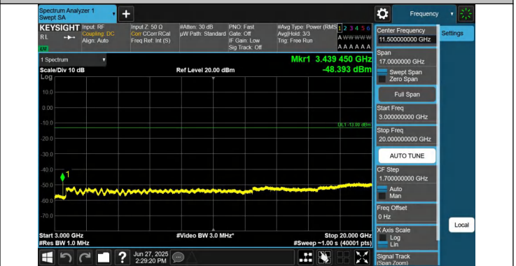
66-66-10MHz-15MHz-QPSK-QPSK-132025-132145-1RB#49-0R B#0-3000~20000MHz-PASS
