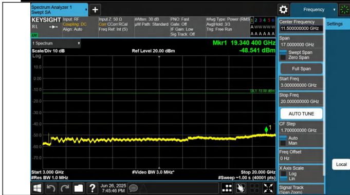
66-66-5MHz-20MHz-QPSK-QPSK-132027-132171-1RB#24-0RB #0-3000~20000MHz-PASS
