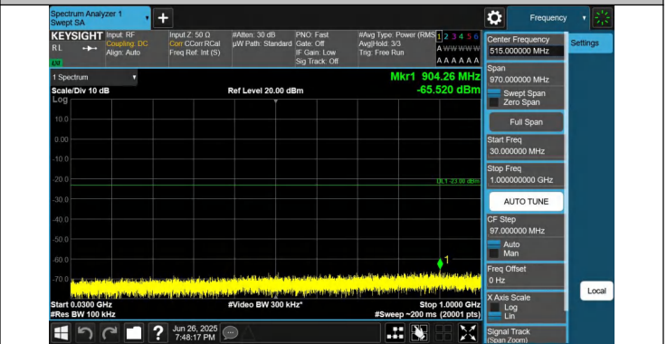
66-66-5MHz-20MHz-QPSK-QPSK-132328-132472-1RB#24-0RB #0-30~1000MHz-PASS
