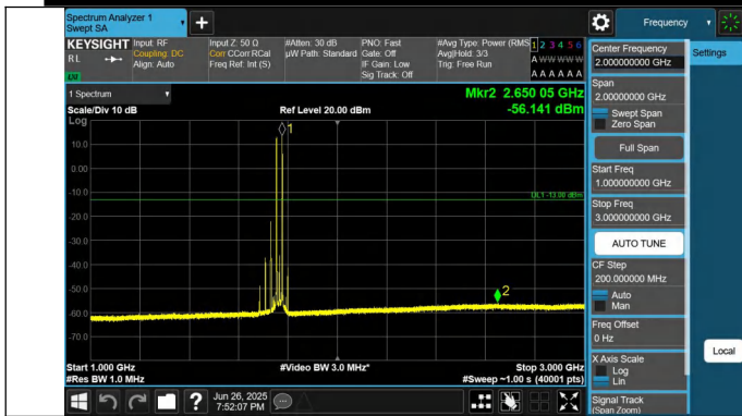
66-66-5MHz-20MHz-QPSK-QPSK-132428-132572-1RB#0-1RB# 99-1000~3000MHz-PASS
