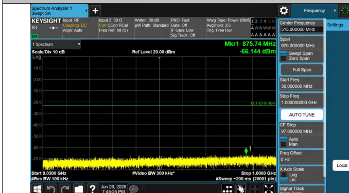
66-66-5MHz-20MHz-QPSK-QPSK-132027-132171-1RB#24-0RB #0-30~1000MHz-PASS
