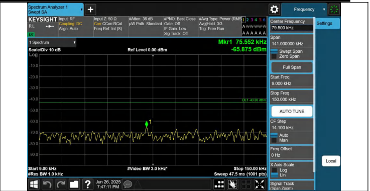
66-66-5MHz-20MHz-QPSK-QPSK-132328-132472-1RB#0-0RB# 0-0.009~0.15MHz-PASS
