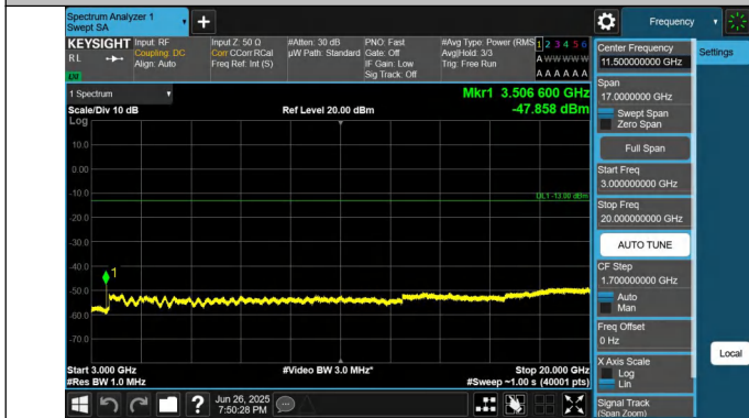
66-66-5MHz-20MHz-QPSK-QPSK-132428-132572-1RB#0-0RB# 0-3000~20000MHz-PASS
