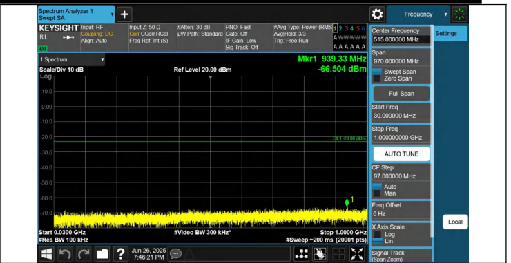
66-66-5MHz-20MHz-QPSK-QPSK-132027-132171-1RB#0-1RB# 99-30~1000MHz-PASS
