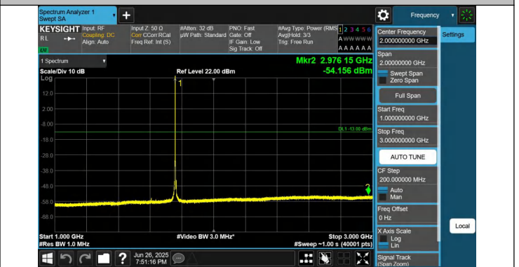
66-66-5MHz-20MHz-QPSK-QPSK-132428-132572-1RB#24-0RB #0-1000~3000MHz-PASS
