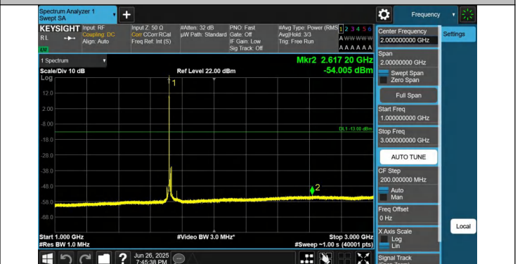
66-66-5MHz-20MHz-QPSK-QPSK-132027-132171-1RB#24-0RB #0-1000~3000MHz-PASS
