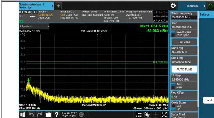
66-66-5MHz-20MHz-QPSK-QPSK-132328-132472-1RB#0-0RB# 0-0.15~30MHz-PASS
