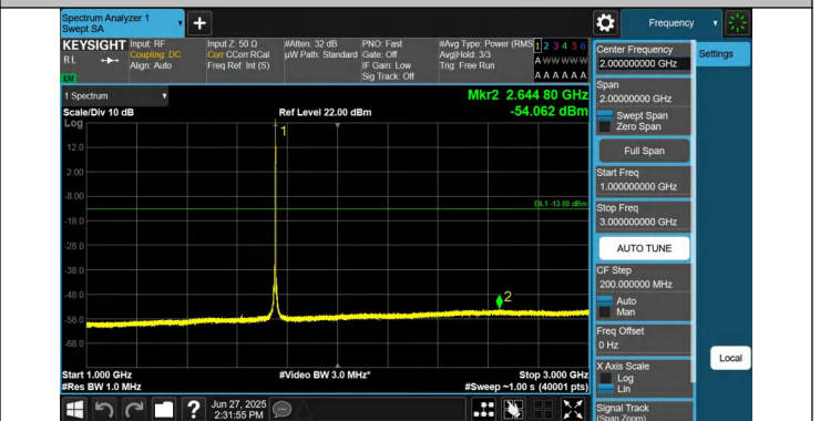
66-66-10MHz-15MHz-QPSK-QPSK-132351-132471-1RB#49-0R B#0-1000~3000MHz-PASS
