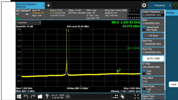
66-66-10MHz-15MHz-QPSK-QPSK-132477-132597-1RB#0-0RB #0-1000~3000MHz-PASS
