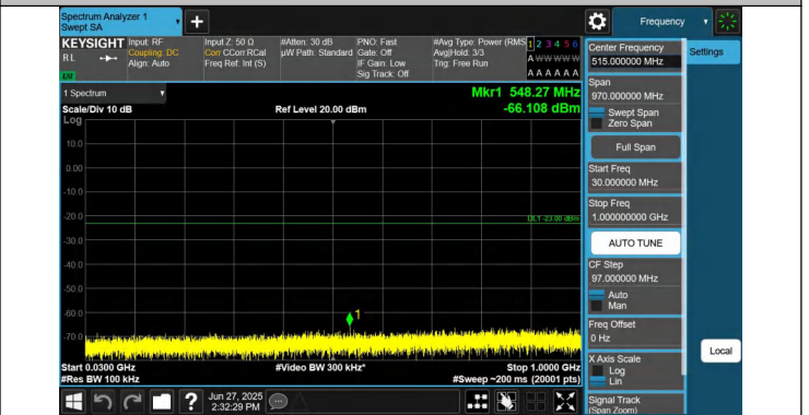
66-66-10MHz-15MHz-QPSK-QPSK-132351-132471-1RB#0-0RB #74-30~1000MHz-PASS
