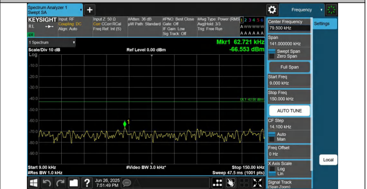
66-66-5MHz-20MHz-QPSK-QPSK-132428-132572-1RB#0-1RB# 99-0.009~0.15MHz-PASS
