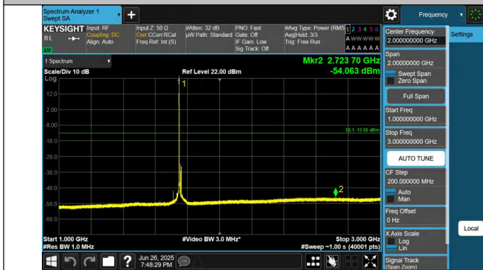
66-66-5MHz-20MHz-QPSK-QPSK-132328-132472-1RB#24-0RB #0-1000~3000MHz-PASS
