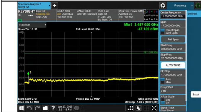
66-66-10MHz-15MHz-QPSK-QPSK-132351-132471-1RB#0-0RB #0-3000~20000MHz-PASS
