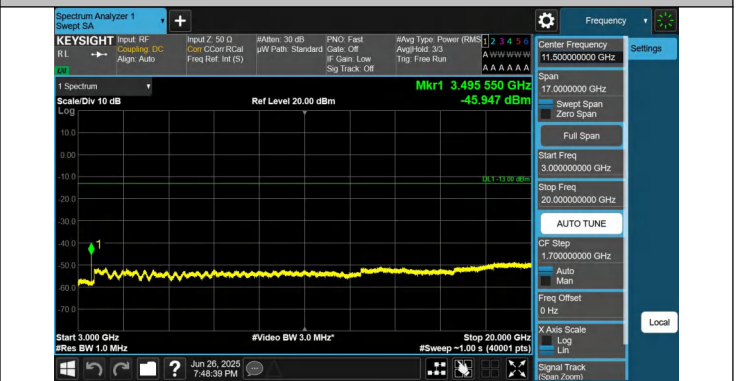
66-66-5MHz-20MHz-QPSK-QPSK-132328-132472-1RB#24-0RB #0-3000~20000MHz-PASS
