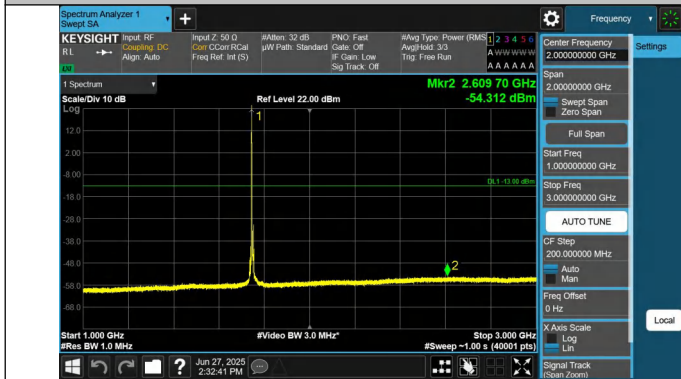
66-66-10MHz-15MHz-QPSK-QPSK-132351-132471-1RB#0-0RB #74-1000~3000MHz-PASS
