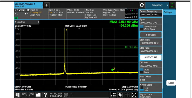
66-66-10MHz-15MHz-QPSK-QPSK-132477-132597-1RB#0-1RB #74-1000~3000MHz-PASS
