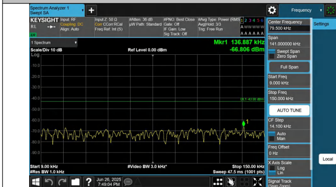
66-66-5MHz-20MHz-QPSK-QPSK-132328-132472-1RB#0-1RB# 99-0.009~0.15MHz-PASS
