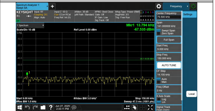
66-66-10MHz-15MHz-QPSK-QPSK-132477-132597-1RB#0-0RB #0-0.009~0.15MHz-PASS
