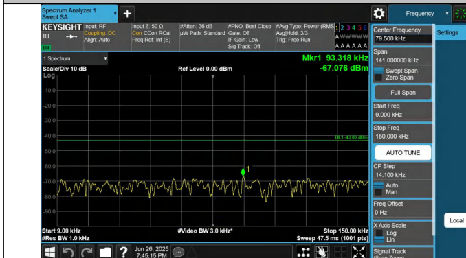
66-66-5MHz-20MHz-QPSK-QPSK-132027-132171-1RB#24-0RB #0-0.009~0.15MHz-PASS
