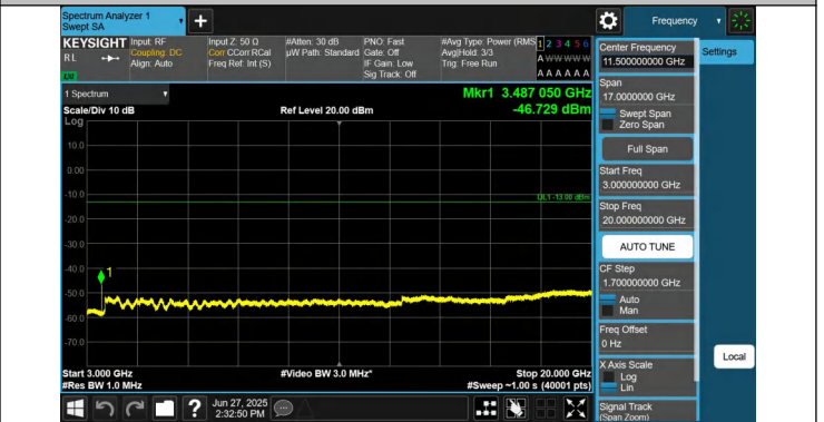
66-66-10MHz-15MHz-QPSK-QPSK-132351-132471-1RB#0-0RB #74-3000~20000MHz-PASS
