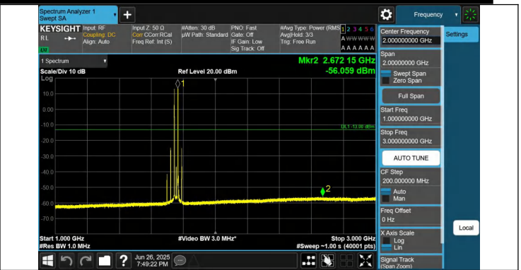
66-66-5MHz-20MHz-QPSK-QPSK-132328-132472-1RB#0-1RB# 99-1000~3000MHz-PASS
