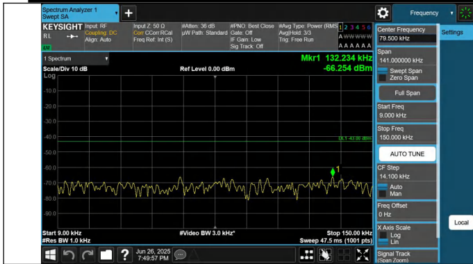
66-66-5MHz-20MHz-QPSK-QPSK-132428-132572-1RB#0-0RB# 0-0.009~0.15MHz-PASS
