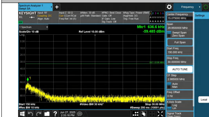
66-66-10MHz-15MHz-QPSK-QPSK-132477-132597-1RB#0-0RB #0-0.15~30MHz-PASS
