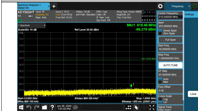
66-66-5MHz-20MHz-QPSK-QPSK-132428-132572-1RB#24-0RB #0-30~1000MHz-PASS
