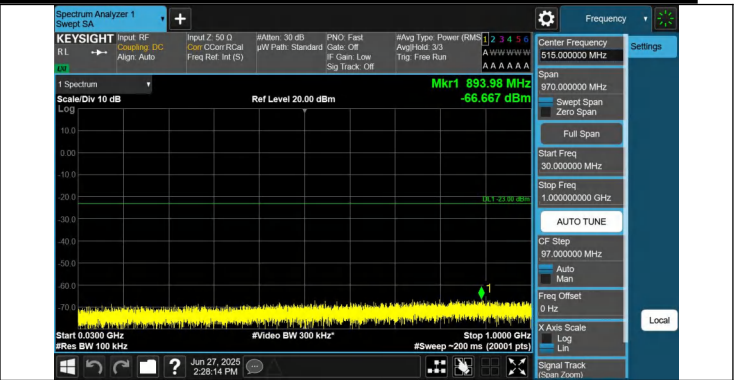
66-66-10MHz-15MHz-QPSK-QPSK-132025-132145-1RB#0-0RB #0-30~1000MHz-PASS
