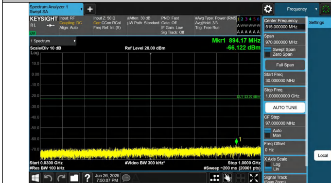
66-66-5MHz-20MHz-QPSK-QPSK-132428-132572-1RB#0-0RB# 0-30~1000MHz-PASS
