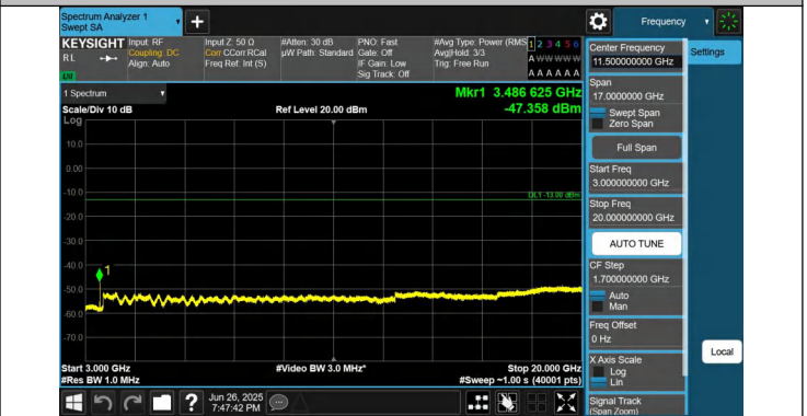
66-66-5MHz-20MHz-QPSK-QPSK-132328-132472-1RB#0-0RB# 0-3000~20000MHz-PASS
