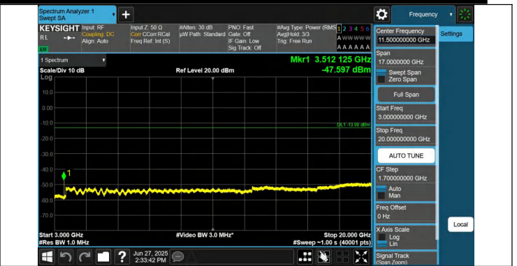
66-66-10MHz-15MHz-QPSK-QPSK-132477-132597-1RB#0-0RB #0-3000~20000MHz-PASS
