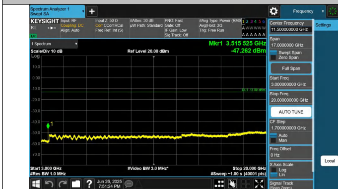
66-66-5MHz-20MHz-QPSK-QPSK-132428-132572-1RB#24-0RB #0-3000~20000MHz-PASS
