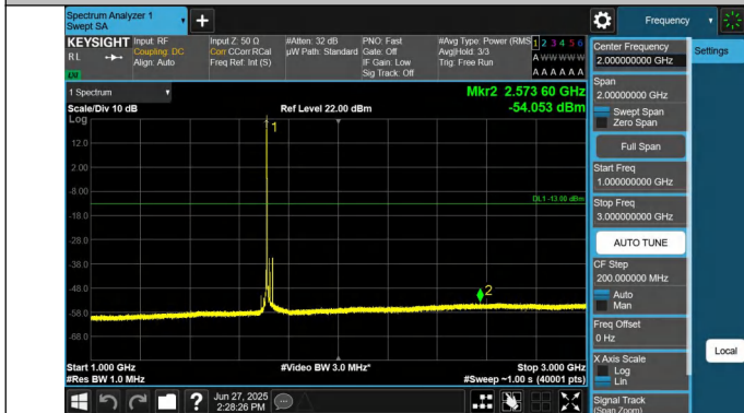
66-66-10MHz-15MHz-QPSK-QPSK-132025-132145-1RB#0-0RB #0-1000~3000MHz-PASS
