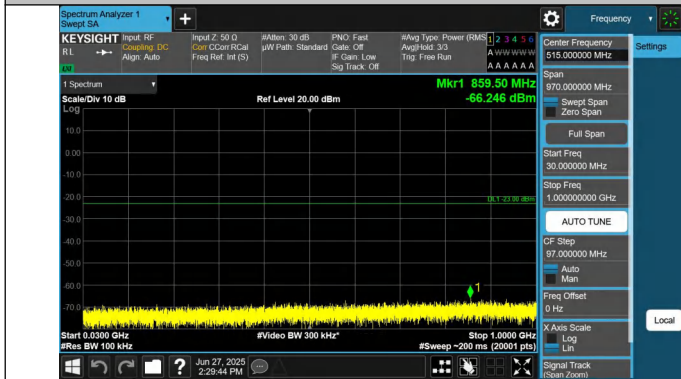
66-66-10MHz-15MHz-QPSK-QPSK-132025-132145-1RB#0-1RB #74-30~1000MHz-PASS
