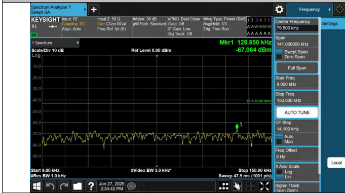
66-66-10MHz-15MHz-QPSK-QPSK-132477-132597-1RB#0-1RB #74-0.009~0.15MHz-PASS
