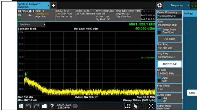
66-66-10MHz-15MHz-QPSK-QPSK-132025-132145-1RB#0-0RB #0-0.15~30MHz-PASS
