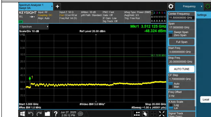
66-66-10MHz-15MHz-QPSK-QPSK-132477-132597-1RB#0-1RB #74-3000~20000MHz-PASS
