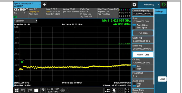
66-66-10MHz-15MHz-QPSK-QPSK-132025-132145-1RB#0-0RB #0-3000~20000MHz-PASS
