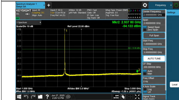
66-66-10MHz-15MHz-QPSK-QPSK-132025-132145-1RB#49-0R B#0-1000~3000MHz-PASS
