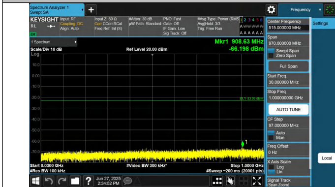
66-66-10MHz-15MHz-QPSK-QPSK-132477-132597-1RB#0-1RB #74-30~1000MHz-PASS
