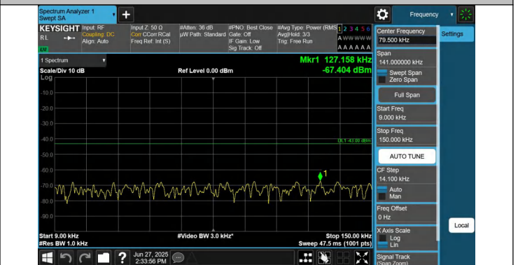
66-66-10MHz-15MHz-QPSK-QPSK-132477-132597-1RB#49-0R B#0-0.009~0.15MHz-PASS
