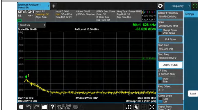
66-66-10MHz-10MHz-QPSK-QPSK-132523-132622-1RB#49-0R B#0-0.15~30MHz-PASS
