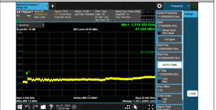
66-66-15MHz-5MHz-QPSK-QPSK-132398-132491-1RB#74-0RB #0-3000~20000MHz-PASS
