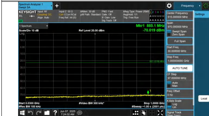
66-66-15MHz-5MHz-QPSK-QPSK-132549-132642-1RB#0-0RB# 0-30~1000MHz-PASS
