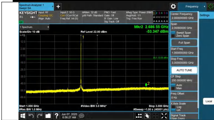
66-66-10MHz-10MHz-QPSK-QPSK-132523-132622-1RB#49-0R B#0-1000~3000MHz-PASS
