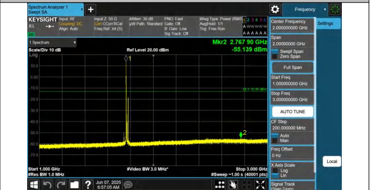
66-66-10MHz-10MHz-QPSK-QPSK-132523-132622-1RB#0-1RB #49-1000~3000MHz-PASS
