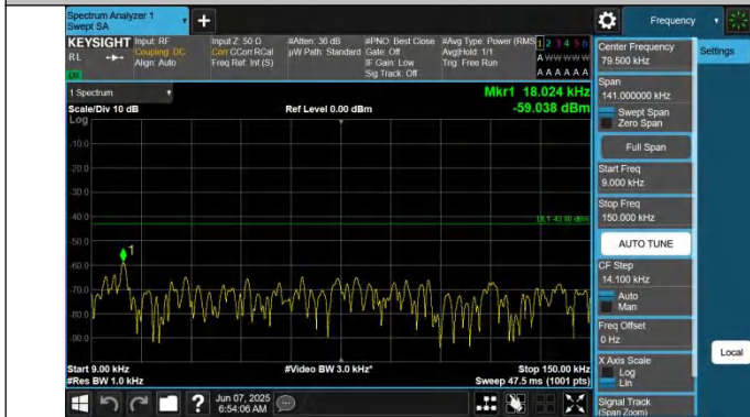
66-66-10MHz-10MHz-QPSK-QPSK-132373-132472-1RB#49-0R B#0-0.009~0.15MHz-PASS
