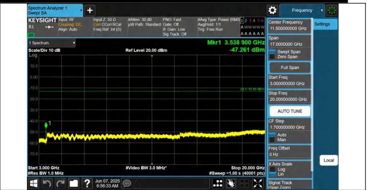
66-66-10MHz-10MHz-QPSK-QPSK-132523-132622-1RB#49-0R B#0-3000~20000MHz-PASS
