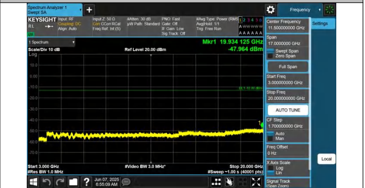
66-66-10MHz-10MHz-QPSK-QPSK-132373-132472-1RB#0-1RB #49-3000~20000MHz-PASS
