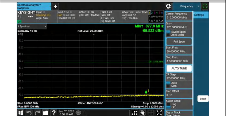
66-66-10MHz-10MHz-QPSK-QPSK-132523-132622-1RB#49-0R B#0-30~1000MHz-PASS
