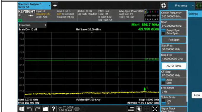
66-66-10MHz-10MHz-QPSK-QPSK-132523-132622-1RB#0-1RB #49-30~1000MHz-PASS
