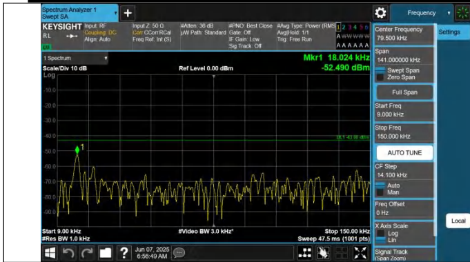
66-66-10MHz-10MHz-QPSK-QPSK-132523-132622-1RB#0-1RB #49-0.009~0.15MHz-PASS
