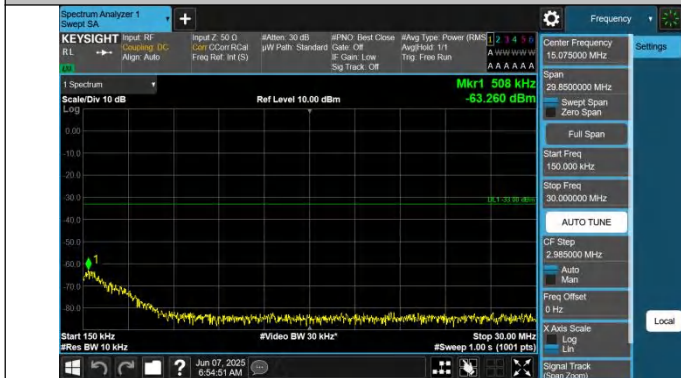
66-66-10MHz-10MHz-QPSK-QPSK-132373-132472-1RB#0-1RB #49-0.15~30MHz-PASS
