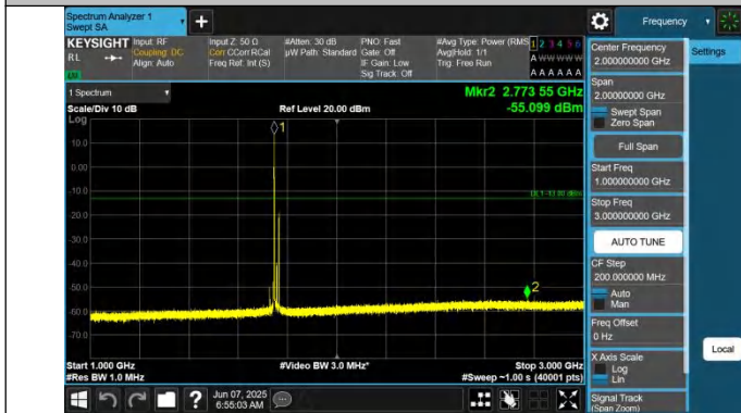
66-66-10MHz-10MHz-QPSK-QPSK-132373-132472-1RB#0-1RB #49-1000~3000MHz-PASS
