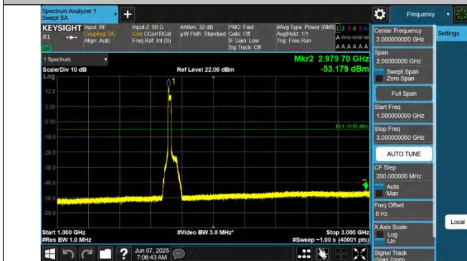
B#0-1000~3000MHz-PASS
