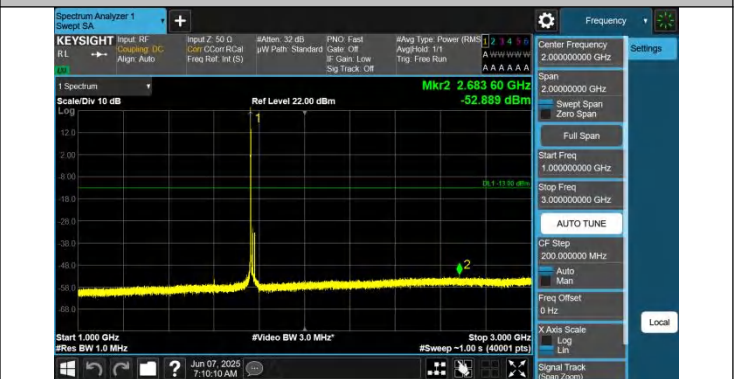
66-66-5MHz-15MHz-QPSK-QPSK-132504-132597-1RB#0-0RB# 0-1000~3000MHz-PASS
