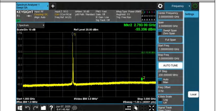
66-66-10MHz-5MHz-QPSK-QPSK-132397-132469-1RB#0-1RB# 24-1000~3000MHz-PASS
