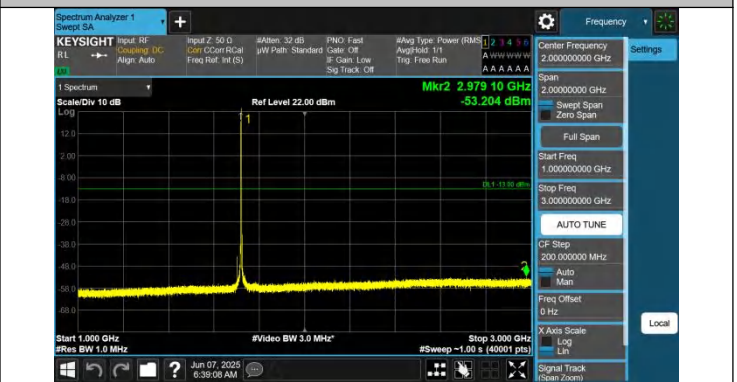
66-66-10MHz-5MHz-QPSK-QPSK-132022-132094-1RB#49-0RB #0-1000~3000MHz-PASS
