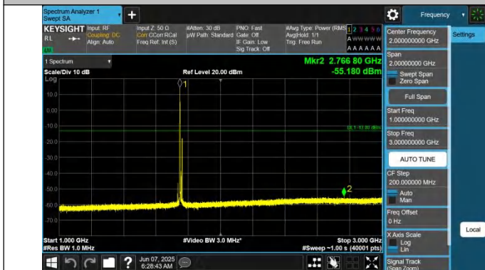
66-66-5MHz-10MHz-QPSK-QPSK-132375-132447-1RB#0-1RB# 49-1000~3000MHz-PASS
