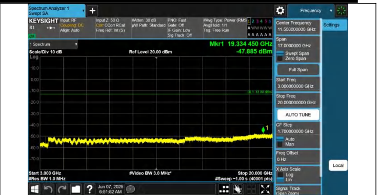
66-66-10MHz-10MHz-QPSK-QPSK-132022-132121-1RB#0-0RB #0-3000~20000MHz-PASS
