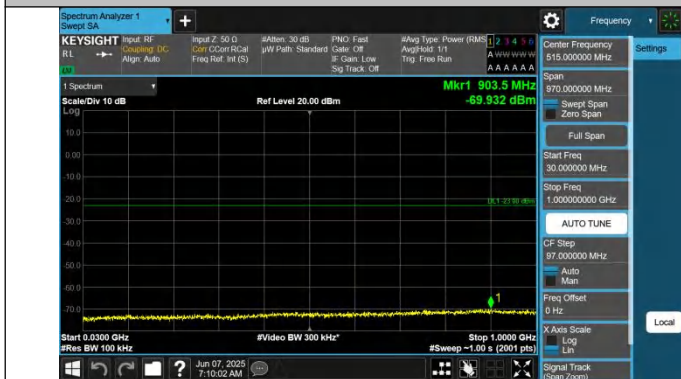
66-66-5MHz-15MHz-QPSK-QPSK-132504-132597-1RB#0-0RB# 0-30~1000MHz-PASS
