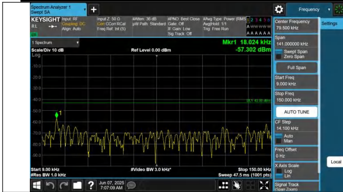
66-66-5MHz-15MHz-QPSK-QPSK-132353-132446-1RB#0-0RB# 0-0.009~0.15MHz-PASS
