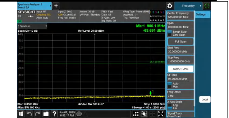
66-66-10MHz-10MHz-QPSK-QPSK-132022-132121-1RB#49-0R B#0-30~1000MHz-PASS
