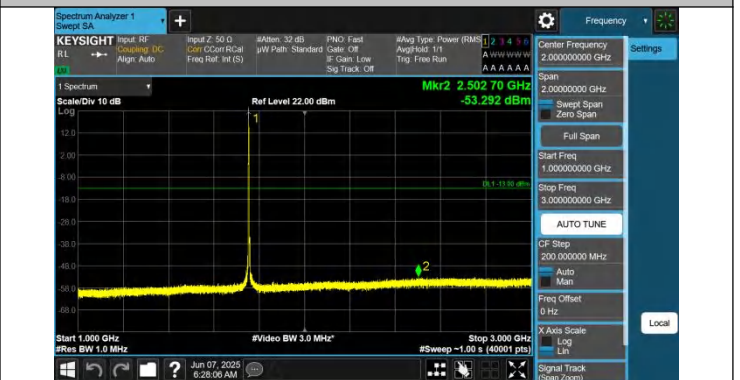
66-66-5MHz-10MHz-QPSK-QPSK-132375-132447-1RB#24-0RB #0-1000~3000MHz-PASS
