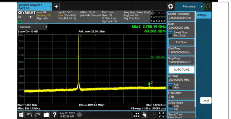
66-66-10MHz-5MHz-QPSK-QPSK-132572-132644-1RB#0-0RB# 0-1000~3000MHz-PASS
