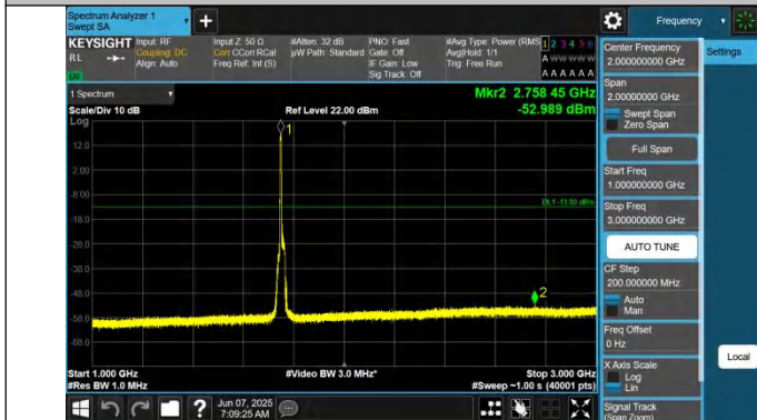
66-66-5MHz-15MHz-QPSK-QPSK-132353-132446-25RB#0-75R B#0-1000~3000MHz-PASS
