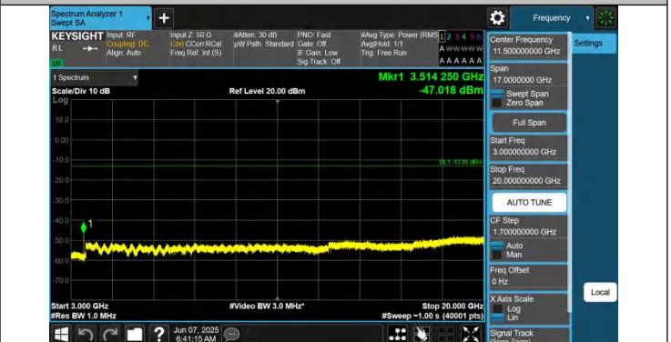
66-66-10MHz-5MHz-QPSK-QPSK-132397-132469-1RB#49-0RB #0-3000~20000MHz-PASS
