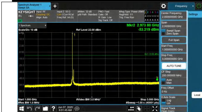
66-66-10MHz-10MHz-QPSK-QPSK-132022-132121-1RB#0-0RB #0-1000~3000MHz-PASS
