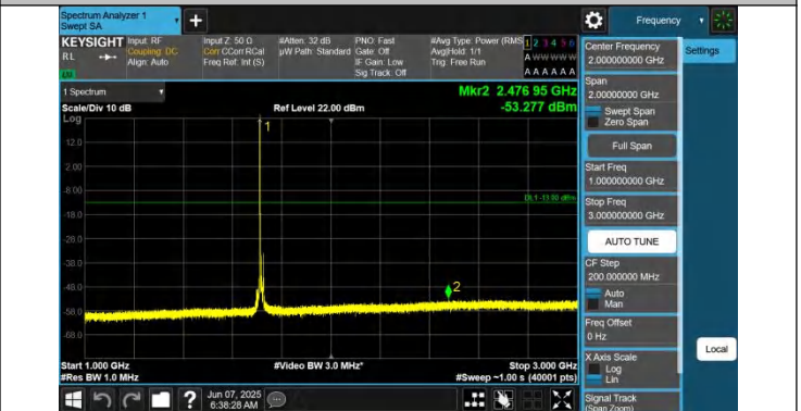
66-66-10MHz-5MHz-QPSK-QPSK-132022-132094-1RB#0-0RB# 0-1000~3000MHz-PASS
