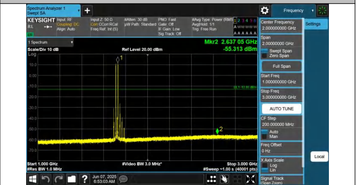
66-66-10MHz-10MHz-QPSK-QPSK-132022-132121-1RB#0-1RB #49-1000~3000MHz-PASS
