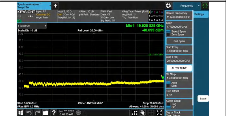
66-66-10MHz-5MHz-QPSK-QPSK-132397-132469-1RB#0-0RB# 0-3000~20000MHz-PASS
