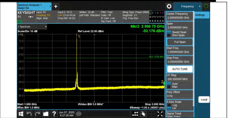
66-66-5MHz-10MHz-QPSK-QPSK-132375-132447-1RB#0-0RB# 0-1000~3000MHz-PASS
