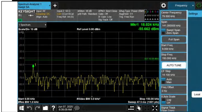
66-66-10MHz-5MHz-QPSK-QPSK-132022-132094-1RB#0-0RB# 0-0.009~0.15MHz-PASS
