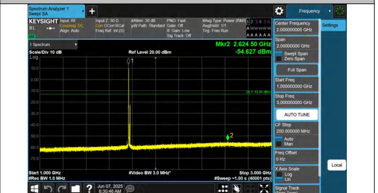
66-66-5MHz-10MHz-QPSK-QPSK-132550-132622-1RB#0-1RB# 49-1000~3000MHz-PASS
