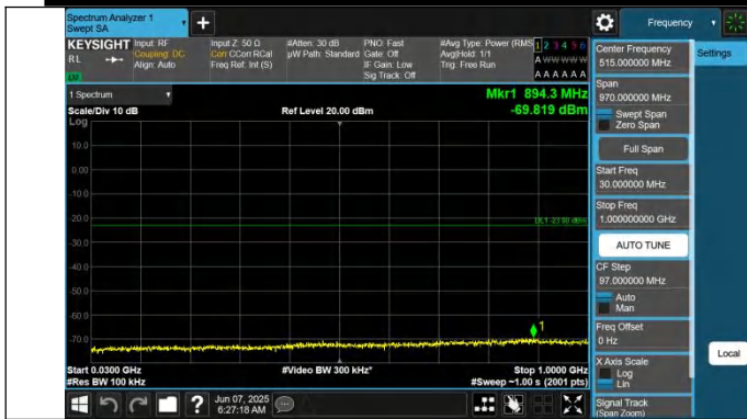
66-66-5MHz-10MHz-QPSK-QPSK-132375-132447-1RB#0-0RB# 0-30~1000MHz-PASS
