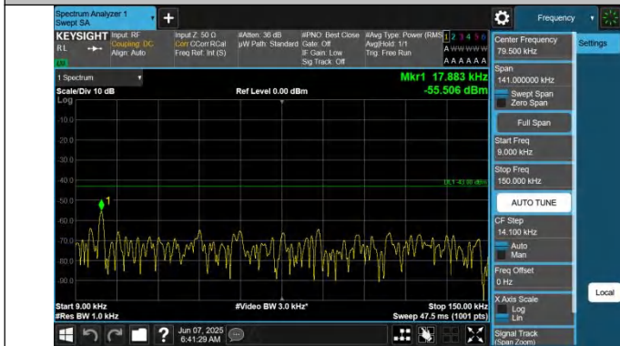
66-66-10MHz-5MHz-QPSK-QPSK-132397-132469-1RB#0-1RB# 24-0.009~0.15MHz-PASS
