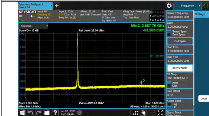
66-66-10MHz-5MHz-QPSK-QPSK-132397-132469-1RB#0-0RB# 0-1000~3000MHz-PASS
