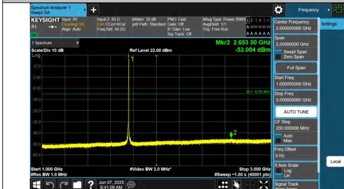
66-66-10MHz-5MHz-QPSK-QPSK-132397-132469-1RB#49-0RB #0-1000~3000MHz-PASS
