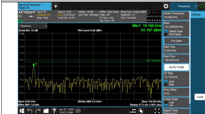
66-66-10MHz-5MHz-QPSK-QPSK-132572-132644-1RB#0-0RB# 0-0.009~0.15MHz-PASS
