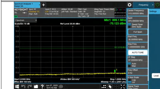
66-66-10MHz-5MHz-QPSK-QPSK-132397-132469-1RB#0-1RB# 24-30~1000MHz-PASS
