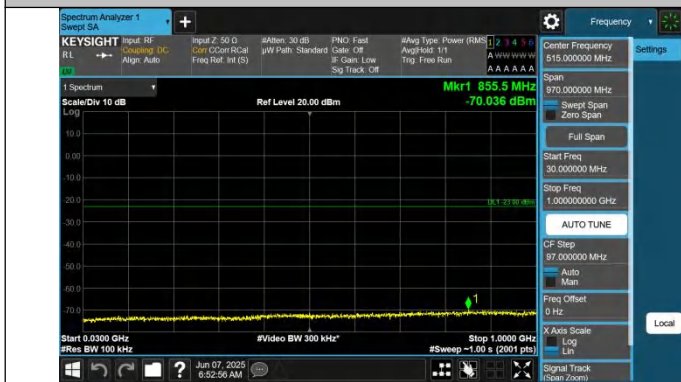
66-66-10MHz-10MHz-QPSK-QPSK-132022-132121-1RB#0-1RB #49-30~1000MHz-PASS
