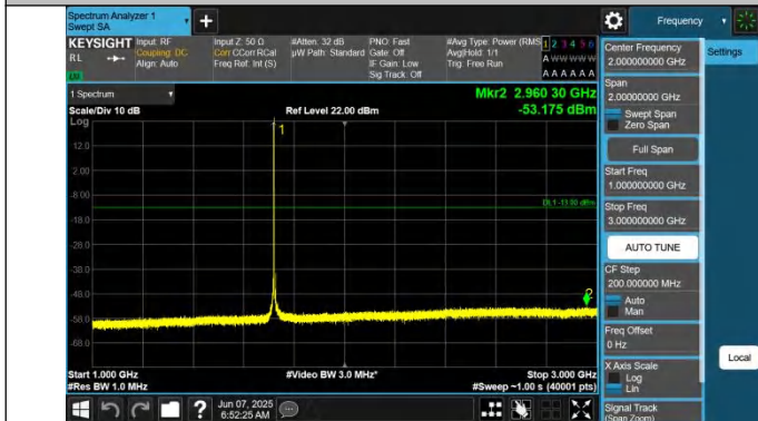
66-66-10MHz-10MHz-QPSK-QPSK-132022-132121-1RB#49-0R B#0-1000~3000MHz-PASS
