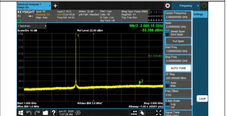
66-66-5MHz-15MHz-QPSK-QPSK-132353-132446-1RB#0-0RB# 0-1000~3000MHz-PASS
