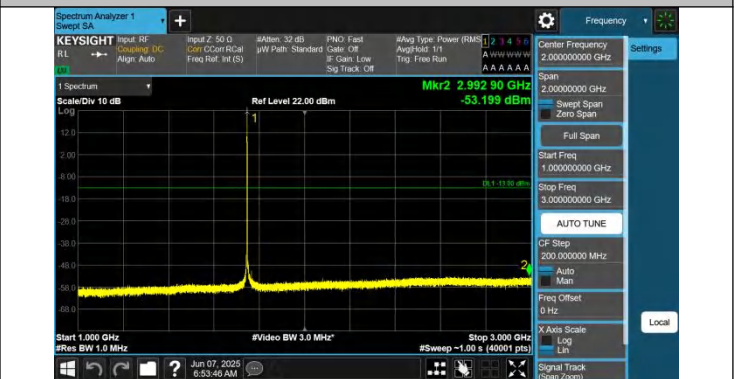
66-66-10MHz-10MHz-QPSK-QPSK-132373-132472-1RB#0-0RB #0-1000~3000MHz-PASS
