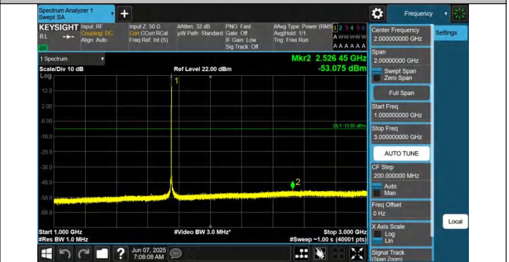
66-66-5MHz-15MHz-QPSK-QPSK-132353-132446-1RB#24-0RB #0-1000~3000MHz-PASS
