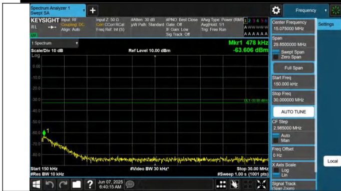
66-66-10MHz-5MHz-QPSK-QPSK-132397-132469-1RB#0-0RB# 0-0.15~30MHz-PASS
