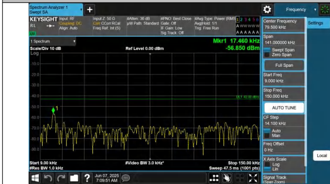
66-66-5MHz-15MHz-QPSK-QPSK-132504-132597-1RB#0-0RB# 0-0.009~0.15MHz-PASS
