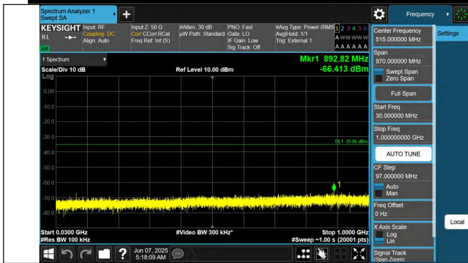
41-41-20MHz-20MHz-QPSK-QPSK-39750-39948-1RB#99-0RB# 0-30~1000MHz-PASS
