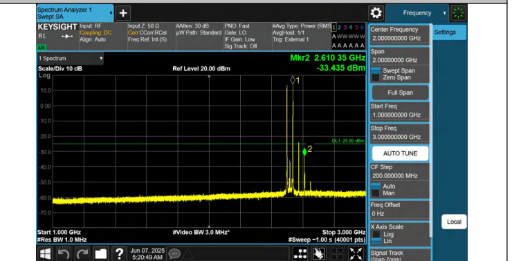
41-41-20MHz-20MHz-QPSK-QPSK-39750-39948-1RB#0-1RB#99 -1000~3000MHz-PASS
