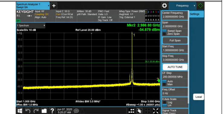
41-41-20MHz-20MHz-QPSK-QPSK-40521-40719-1RB#99-0RB#0 -1000~3000MHz-PASS
