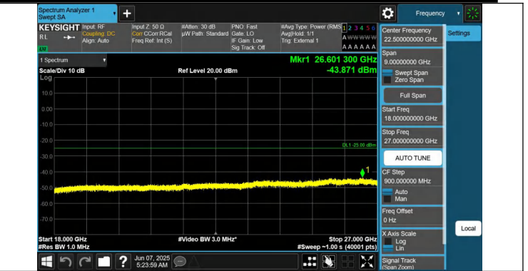
41-41-20MHz-20MHz-QPSK-QPSK-40521-40719-1RB#0-0RB#0-18000~27000MHz-PASS
