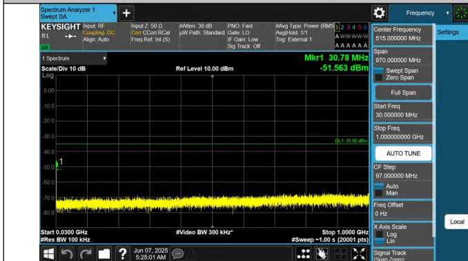
41-41-20MHz-20MHz-QPSK-QPSK-40521-40719-1RB#99-0RB# 0-30~1000MHz-PASS
