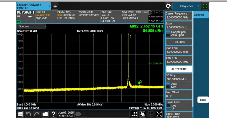
41-41-20MHz-20MHz-QPSK-QPSK-39750-39948-1RB#0-0RB#0- 1000~3000MHz-PASS
