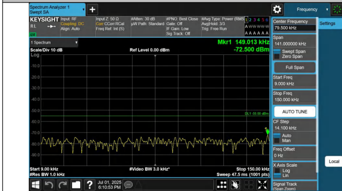
41-41-20MHz-20MHz-QPSK-QPSK-39750-39948-1RB#99-0RB# 0-0.009~0.15MHz-PASS
