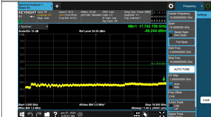
41-41-20MHz-20MHz-QPSK-QPSK-40521-40719-1RB#99-0RB# 0-3000~18000MHz-PASS
