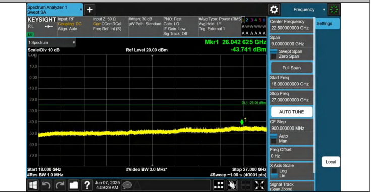
41-41-20MHz-15MHz-QPSK-QPSK-41341-41512-1RB#0-1RB#74 -18000~27000MHz-PASS
