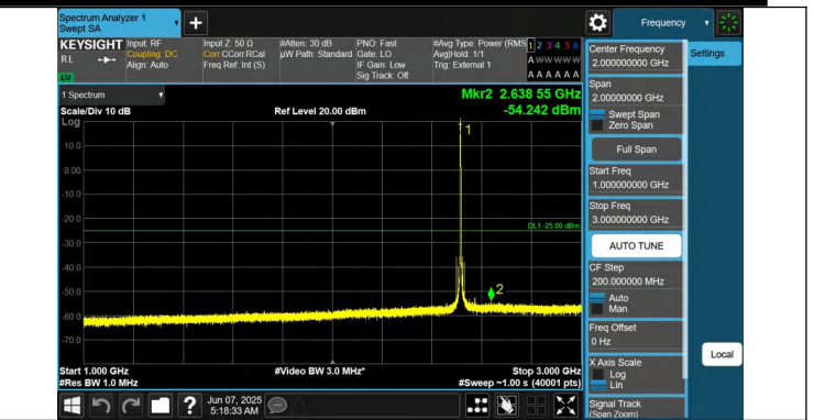
41-41-20MHz-20MHz-QPSK-QPSK-39750-39948-1RB#99-0RB#0 -1000~3000MHz-PASS
