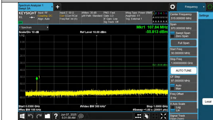
41-41-20MHz-20MHz-QPSK-QPSK-41292-41490-1RB#99-0RB# 0-30~1000MHz-PASS
