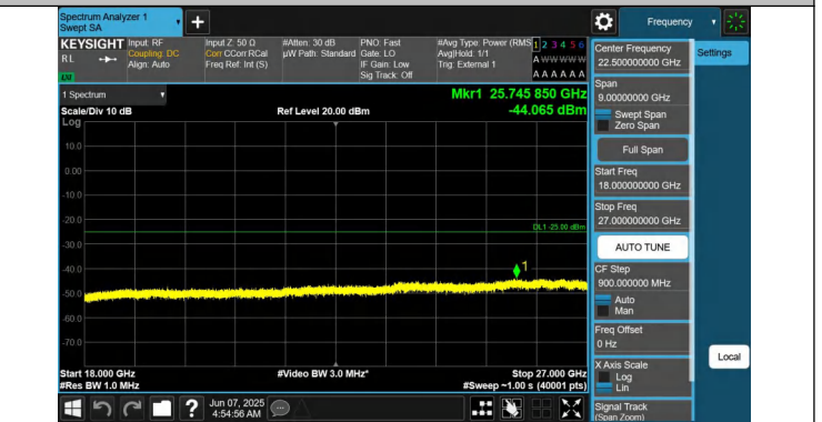
41-41-20MHz-15MHz-QPSK-QPSK-41341-41512-1RB#0-0RB#0- 18000~27000MHz-PASS
