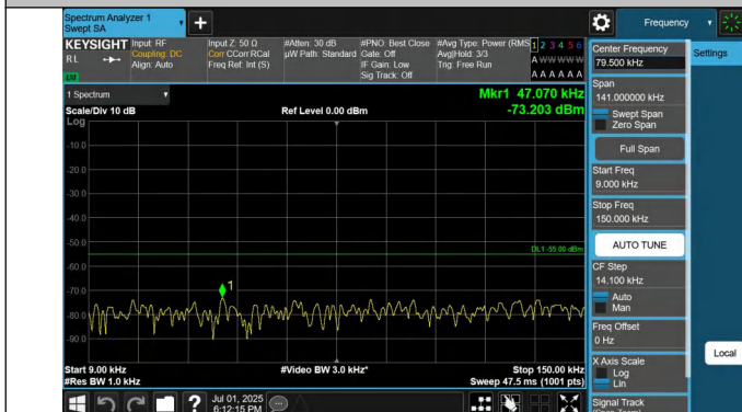
41-41-20MHz-20MHz-QPSK-QPSK-41292-41490-1RB#0-0RB#0- 0.009~0.15MHz-PASS
