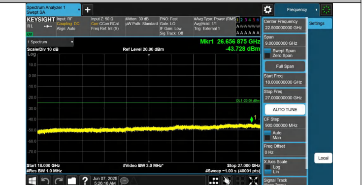
41-41-20MHz-20MHz-QPSK-QPSK-40521-40719-1RB#99-0RB#0 -18000~27000MHz-PASS
