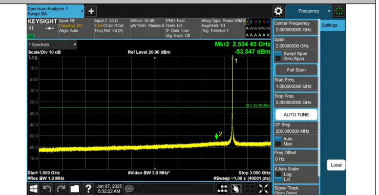
41-41-20MHz-20MHz-QPSK-QPSK-41292-41490-1RB#99-0RB#0 -1000~3000MHz-PASS
