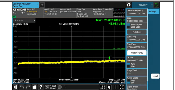
41-41-20MHz-20MHz-QPSK-QPSK-41292-41490-1RB#99-0RB#0 -18000~27000MHz-PASS
