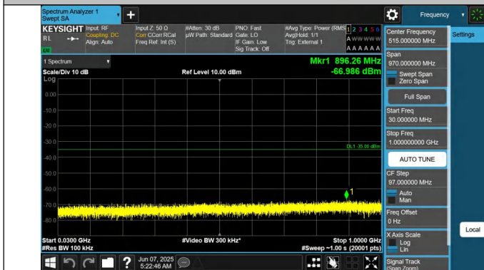
41-41-20MHz-20MHz-QPSK-QPSK-40521-40719-1RB#0-0RB#0- 30~1000MHz-PASS
