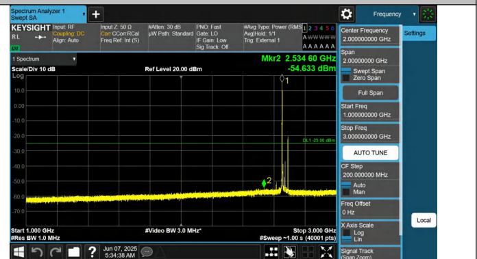
41-41-20MHz-20MHz-QPSK-QPSK-41292-41490-1RB#0-1RB#99-1000~3000MHz-PASS
