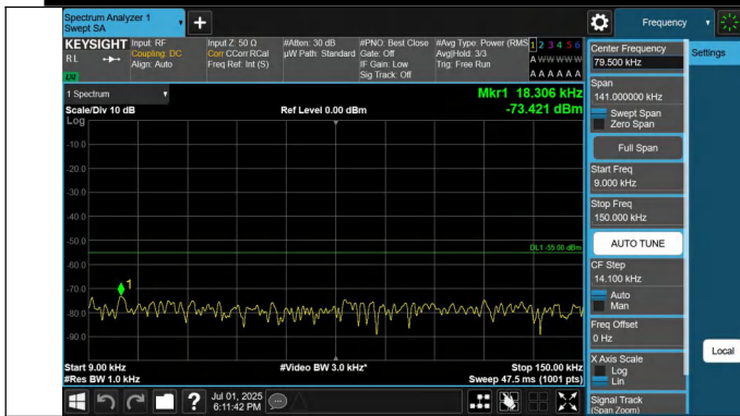
41-41-20MHz-20MHz-QPSK-QPSK-40521-40719-1RB#99-0RB# 0-0.009~0.15MHz-PASS
