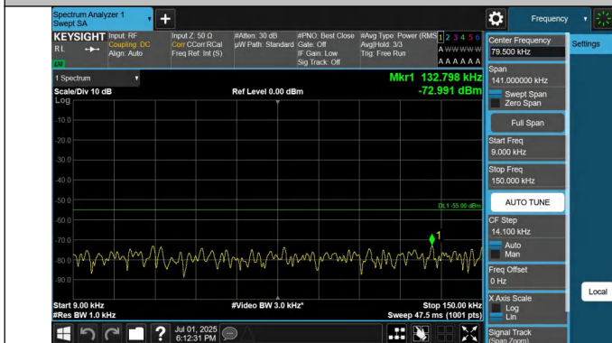
41-41-20MHz-20MHz-QPSK-QPSK-41292-41490-1RB#99-0RB# 0-0.009~0.15MHz-PASS
