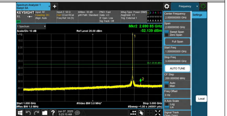
41-41-20MHz-20MHz-QPSK-QPSK-40521-40719-1RB#0-0RB#0- 1000~3000MHz-PASS
