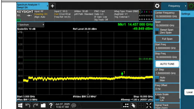
41-41-20MHz-20MHz-QPSK-QPSK-41292-41490-1RB#99-0RB# 0-3000~18000MHz-PASS
