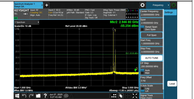
41-41-20MHz-20MHz-QPSK-QPSK-40521-40719-1RB#0-1RB#99-1000~3000MHz-PASS
