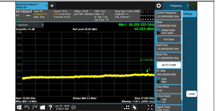
41-41-20MHz-5MHz-QPSK-QPSK-39750-39867-1RB#0-0RB#0-18000~27000MHz-PASS
