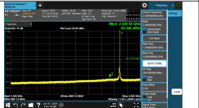
41-41-20MHz-5MHz-QPSK-QPSK-41440-41557-1RB#99-0RB#0- 1000~3000MHz-PASS
