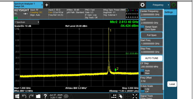
41-41-20MHz-5MHz-QPSK-QPSK-39750-39867-1RB#0-0RB#0-1000~3000MHz-PASS
