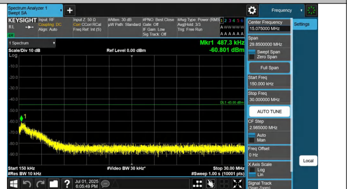
41-41-20MHz-10MHz-QPSK-QPSK-39750-39894-1RB#0-0RB#0- 0.15~30MHz-PASS
