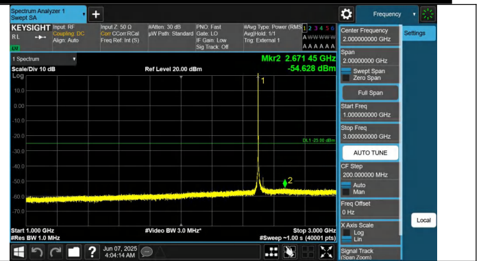
41-41-20MHz-10MHz-QPSK-QPSK-39750-39894-1RB#0-0RB#0-1000~3000MHz-PASS
