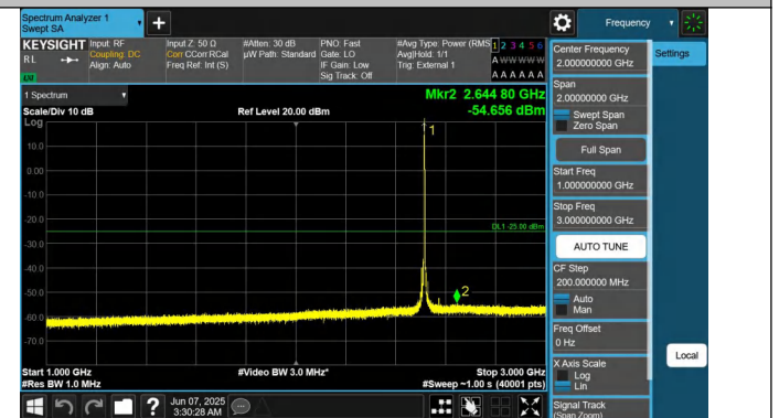
41-41-20MHz-5MHz-QPSK-QPSK-39750-39867-1RB#99-0RB#0-1000~3000MHz-PASS
