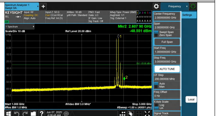
41-41-20MHz-10MHz-QPSK-QPSK-39750-39894-1RB#0-1RB#49-1000~3000MHz-PASS
