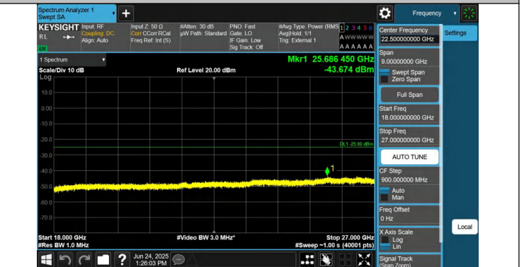
-18000~27000MHz-PASS
