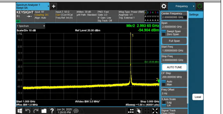
1000~3000MHz-PASS
