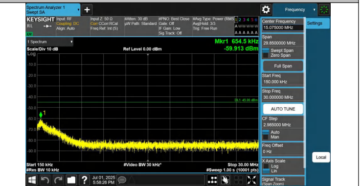
0.15~30MHz-PASS
