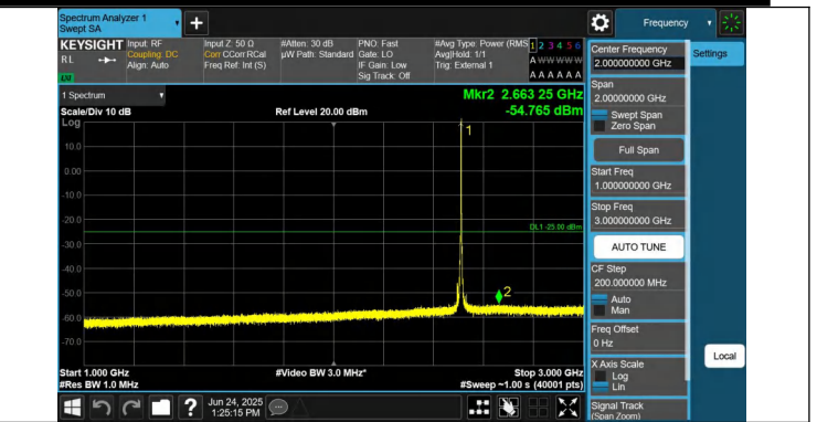
-1000~3000MHz-PASS
