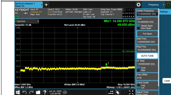
0-3000~18000MHz-PASS
