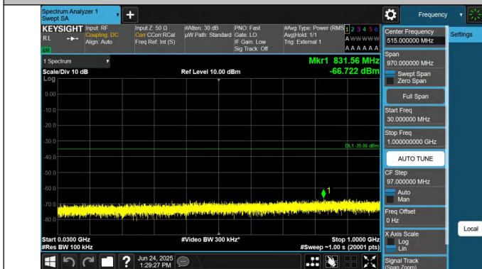
30~1000MHz-PASS
