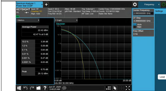
41-41-20MHz-10MHz-QPSK-QPSK-40571-40715-100RB#0-50RB#0-PASS
